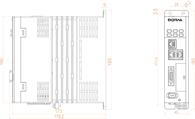
A 机箱： DS3 □ -02AS DS3 □ -04AS
