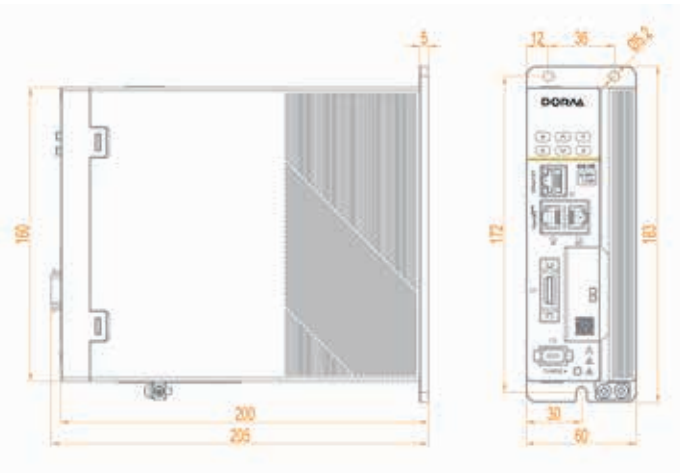
C 机箱： DS3 □ -10BS DS3 □ -15BS
