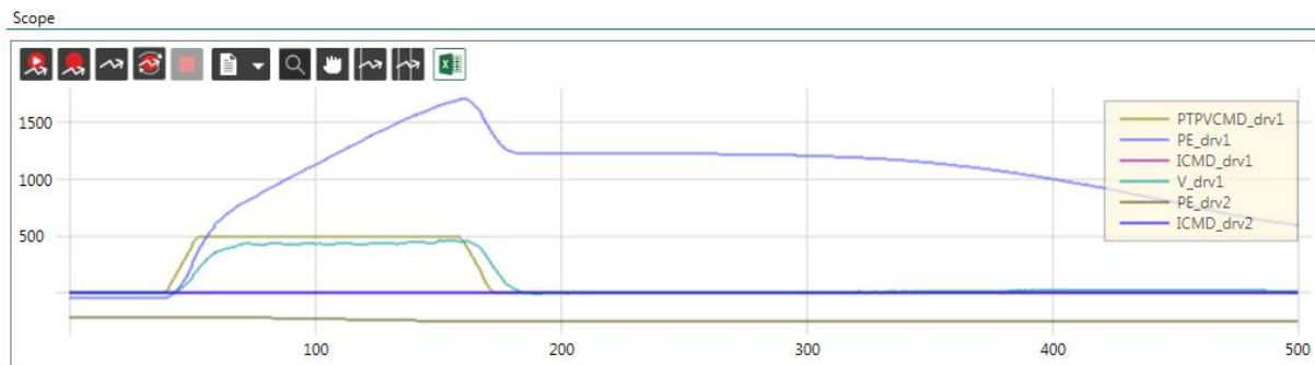
图 8-44 KNLD=1
