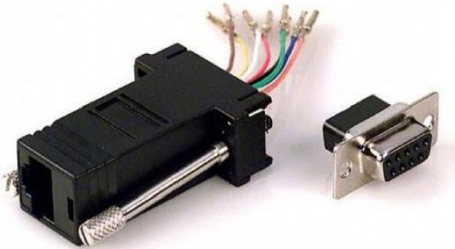
图 11-1 DB9-RJ45 适配器
