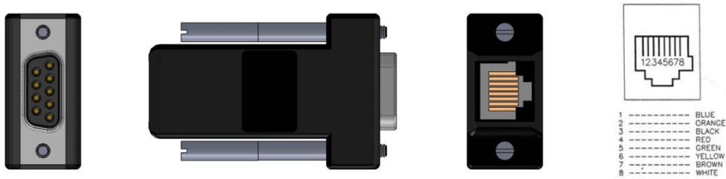
图 11-2 DB9-RJ45 适配器接口
