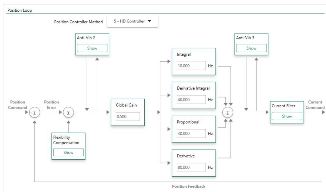
图 7-6 位置控制回路—HD 控制器
