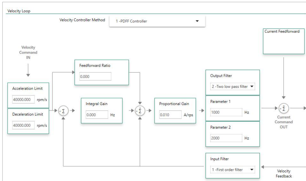
图 7-4 速度控制回路 PDFF 控制器
