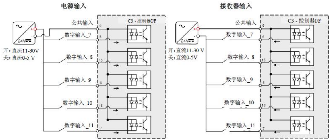
图 4-25 数字输入接线-C3
