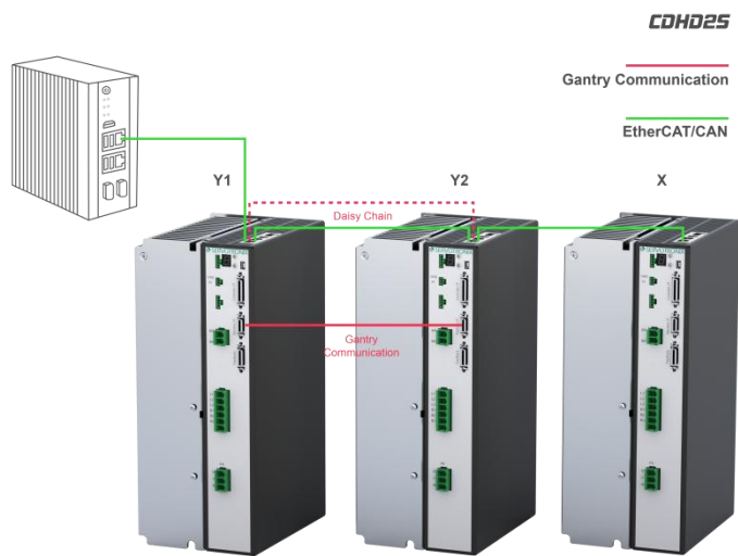
图 4-29 龙门系统接线–EtherCAT/CAN
