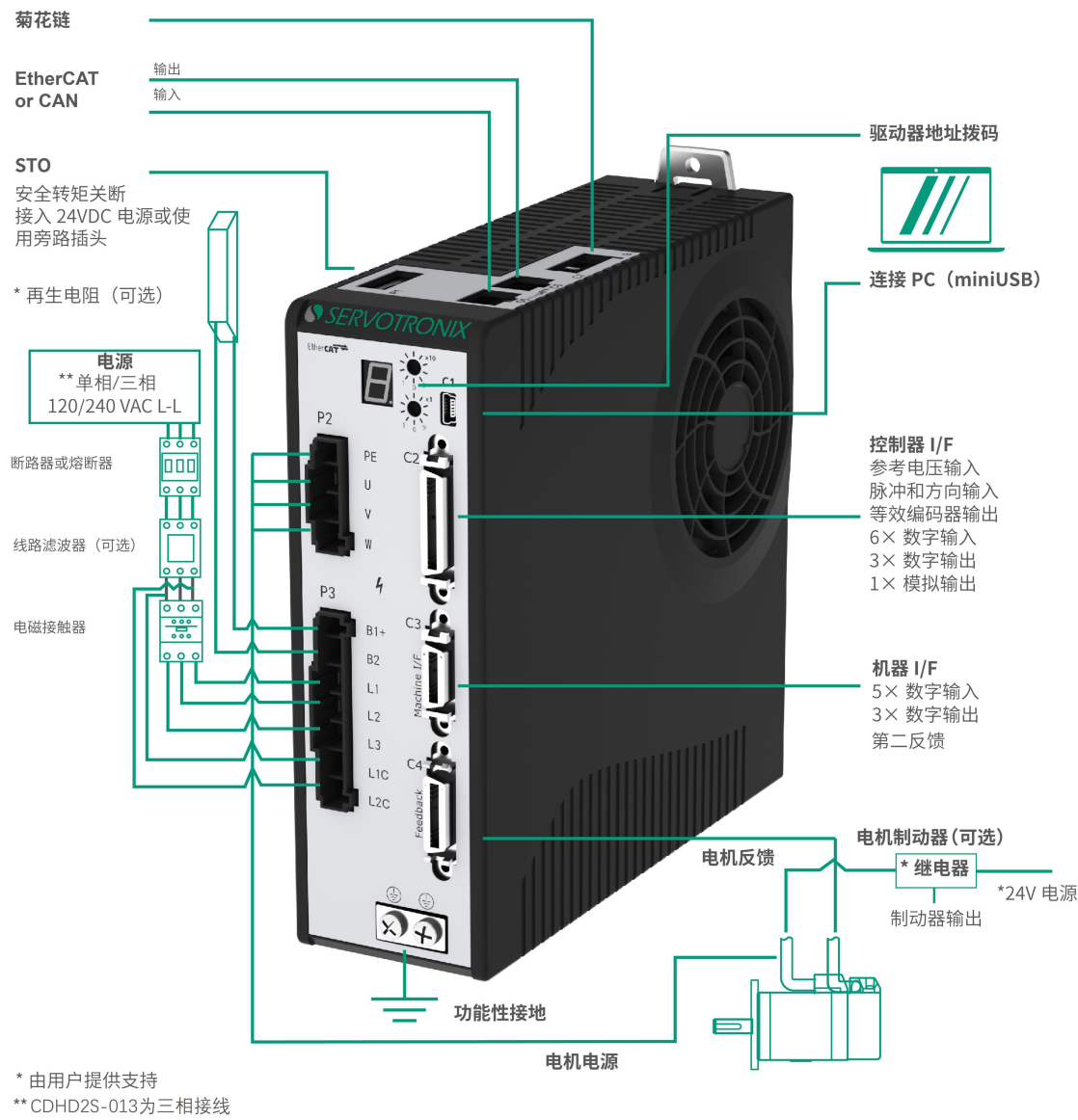
图 4-4 CDHD2S-008/CDHD2S-010/CDHD2S-013 交流 120-240V(中压 EC, AP 及 EC-RO)型号系统接线
