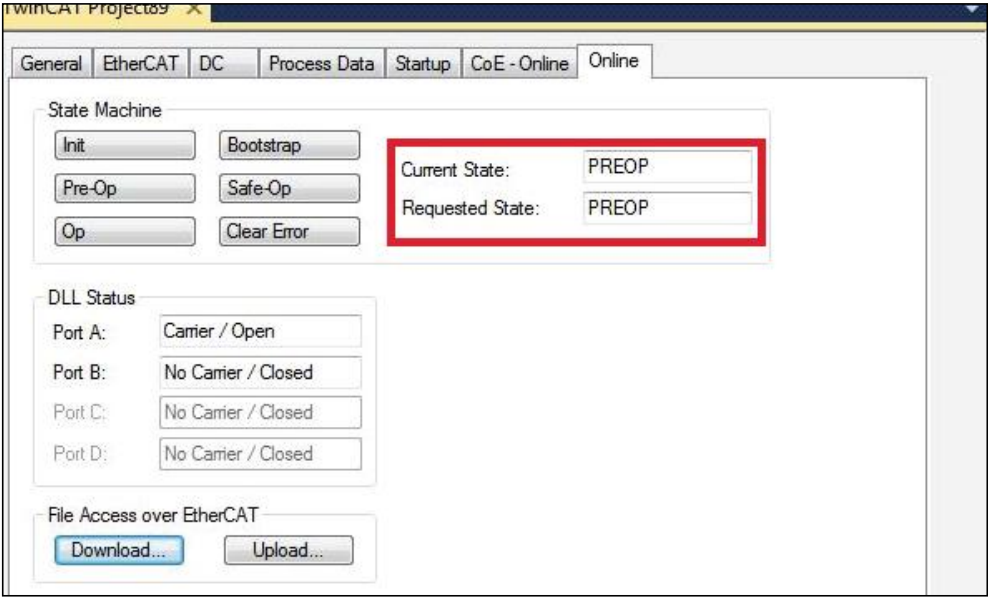
图 4-56 固件更新完成后的当前状态
