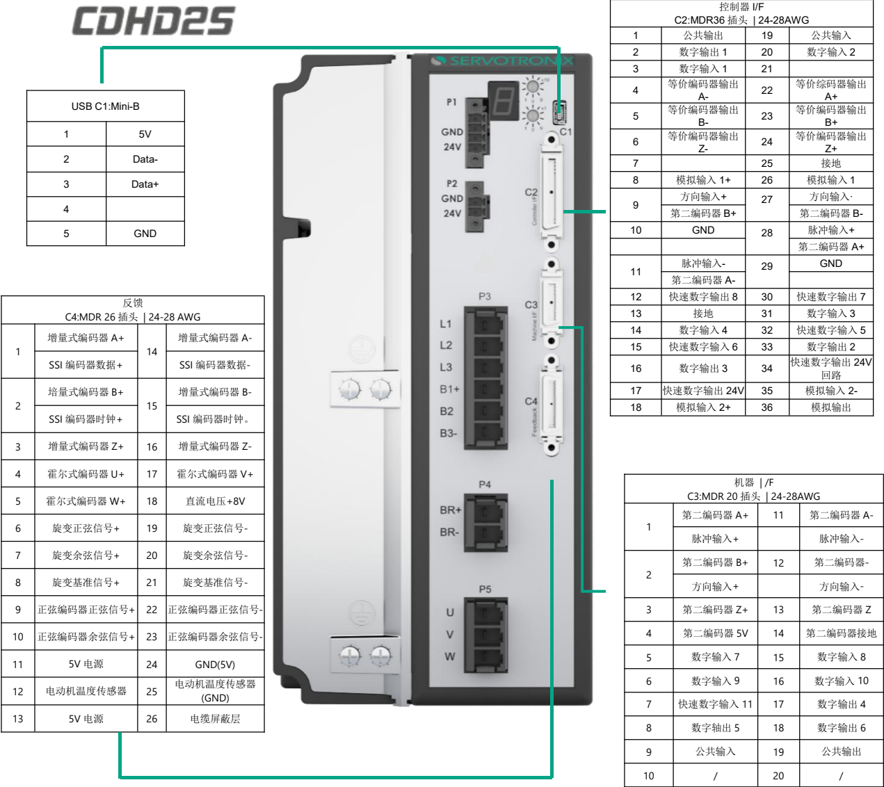
图 4-15 CDHD25 高压 EC 型号控制板引脚分配
