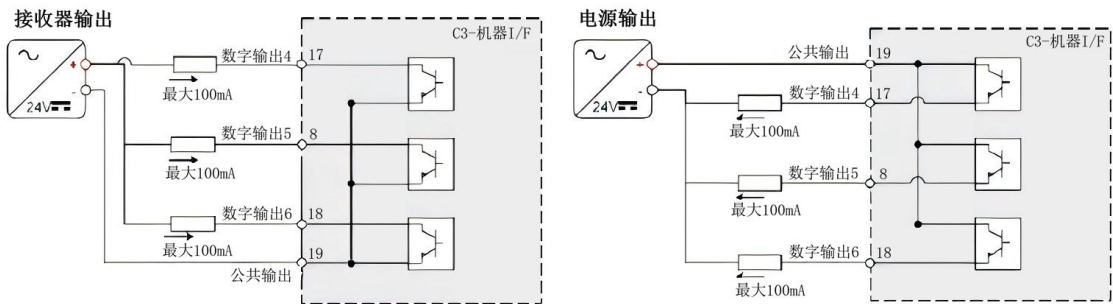
图 4-26 数字输出接线-C3
