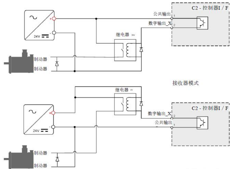
图 4-27 电机制动器接线 CDHD2S(中压型号)
