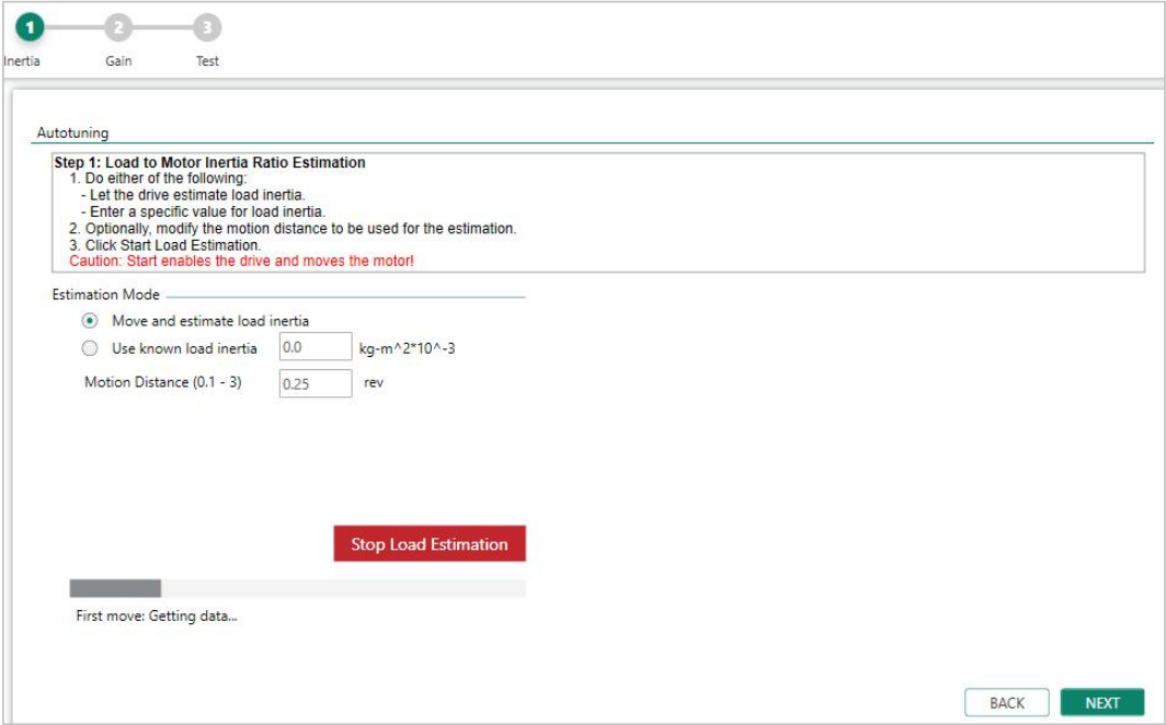
图 8-11 基于 PC 的自动调谐向导——负载/电机惯量比(LMJR)估算
