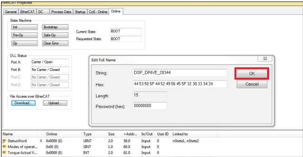
图 4-53 “编辑 FoE 名称”对话框
