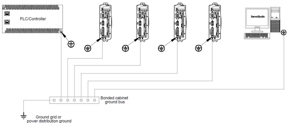
图 4-11 CDHD2S 系统接地
