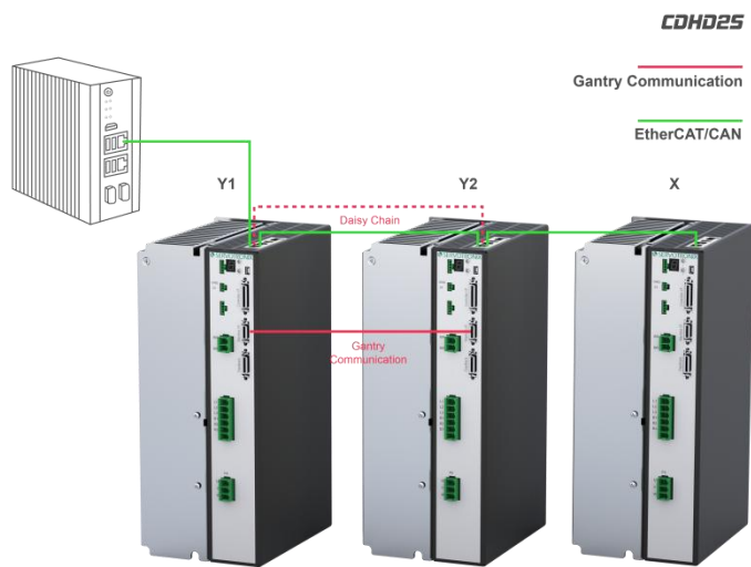
图 4-29 龙门系统接线–EtherCAT/CAN
