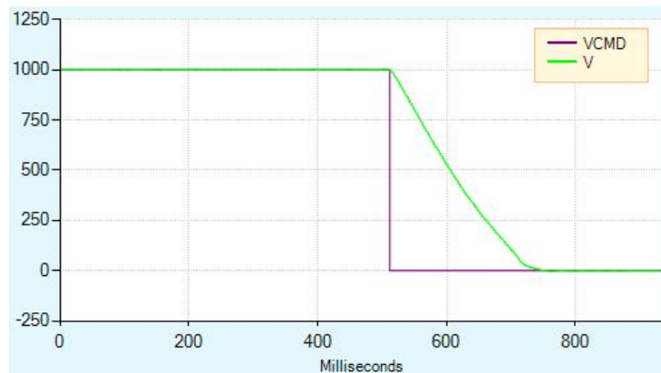
图 6-35 动态制动(低 ISTOP 值)
