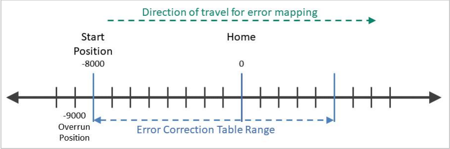
图 6-39 位置补偿映射——示例
