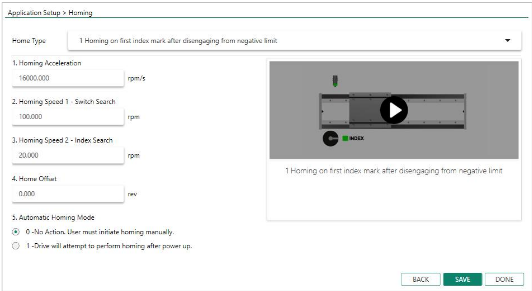
图 6-15 ServoStudio2-应用设置-回零
