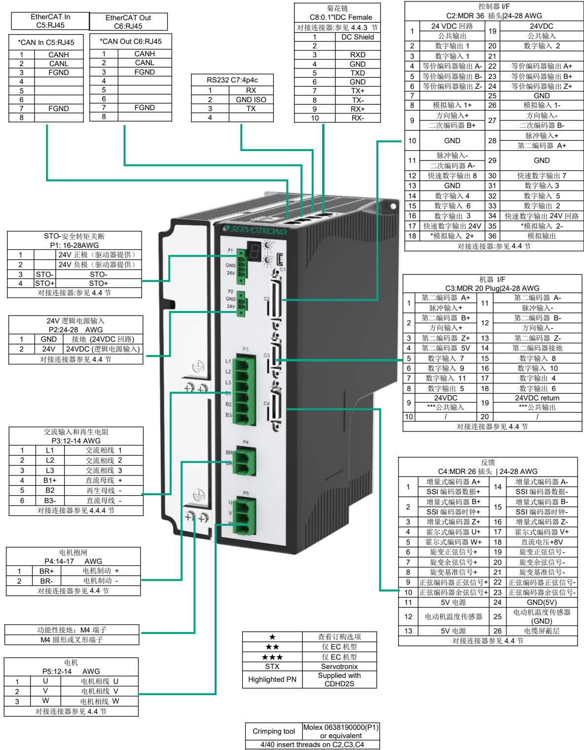
图 4-36 CDHD2S-012(高压)功率板引脚分配
