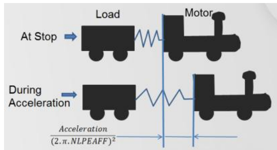
图 8-39 设备柔性
