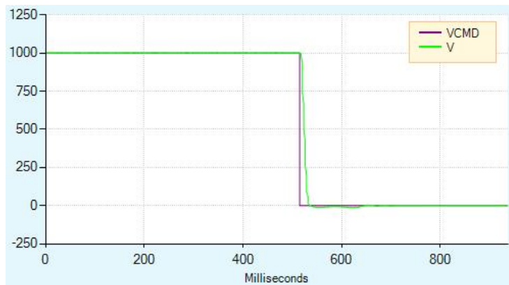
图 6-34 动态制动
