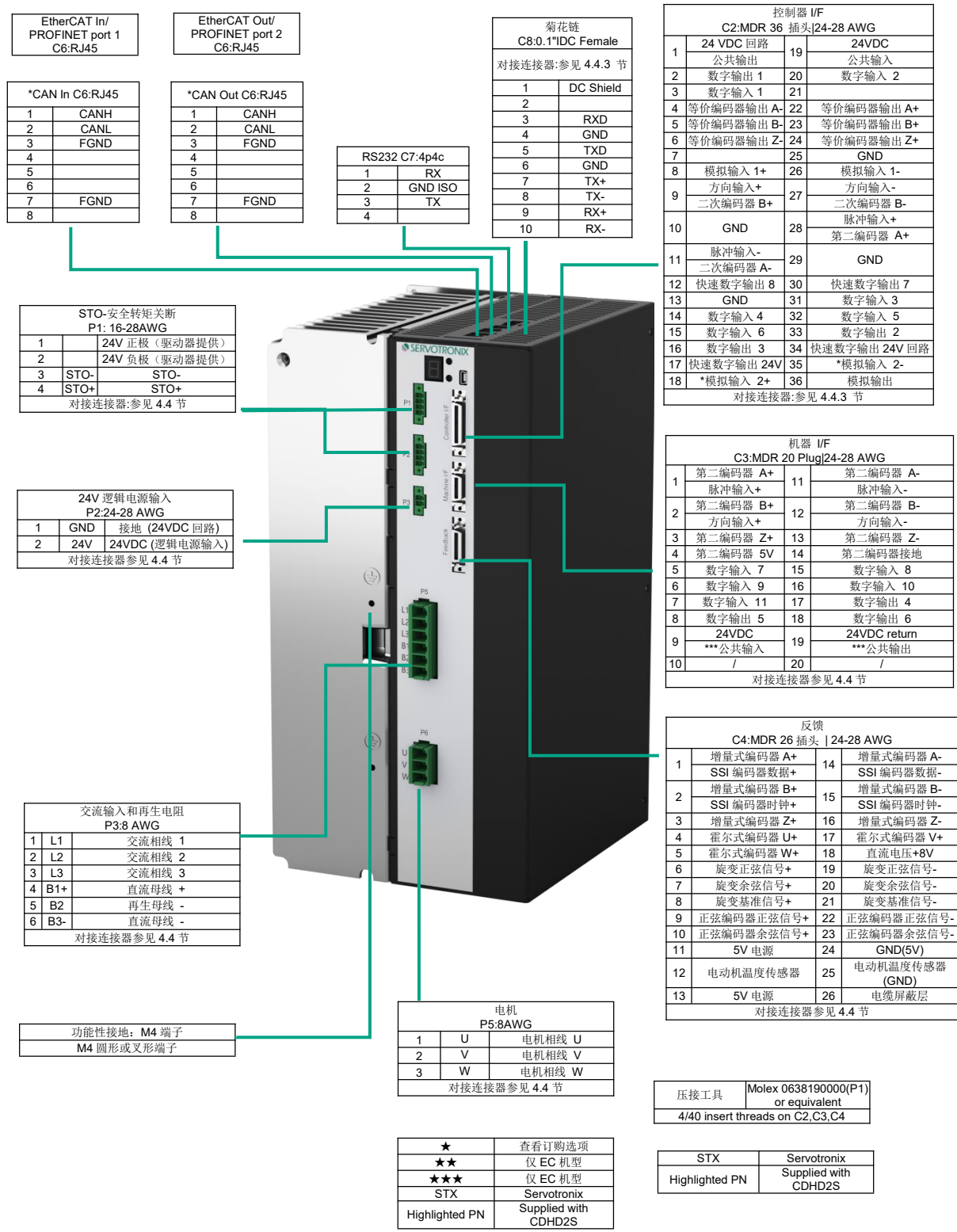
图 4-38 CDHD2S-040(高压)功率板引脚分配
