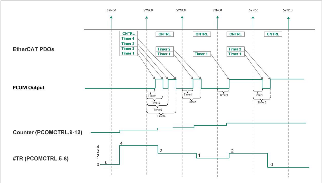
图 6-25 比较匹配触发器输出—定时配置
