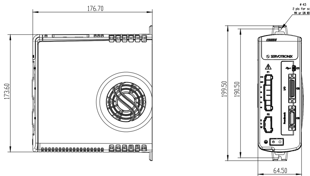
图 3-3 CDHDE-0102AEB 尺寸 (mm)
