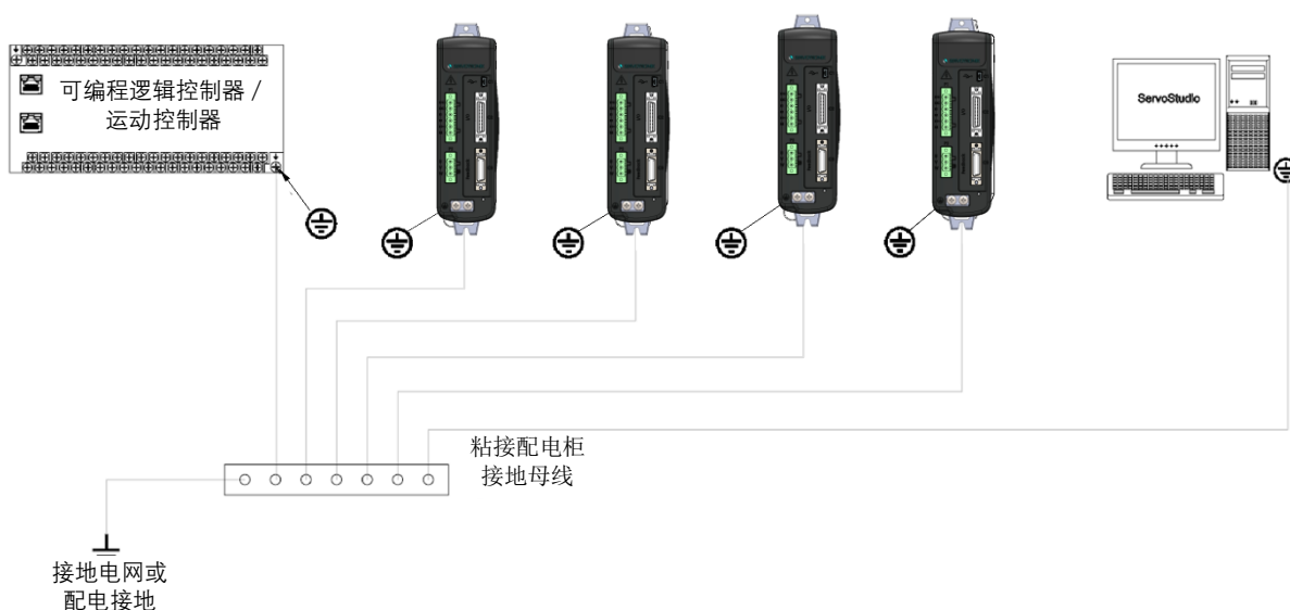
图 4 - 3. CDHDE 系统接地
