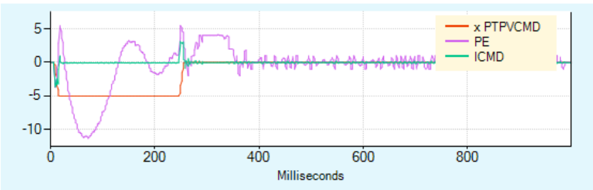
图 8 - 8-6. ICMD 和 PE 效果不佳
