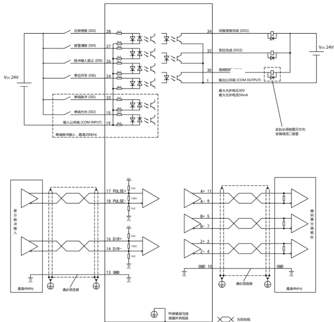
图 4 - 8. CDHDE-0102AAP 默认 IO 接线图
