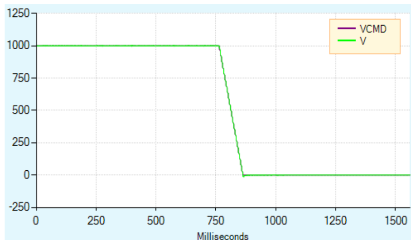
图 6 - 6-8. 禁用（使用活跃禁用）
