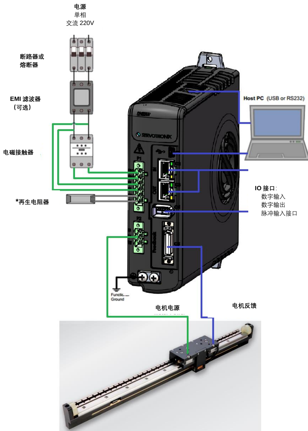
图 4-2 CDHDE-4D52AEB 伺服系统接线
