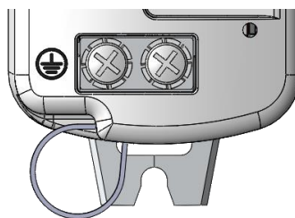
图 4 - 11. 接地端子
