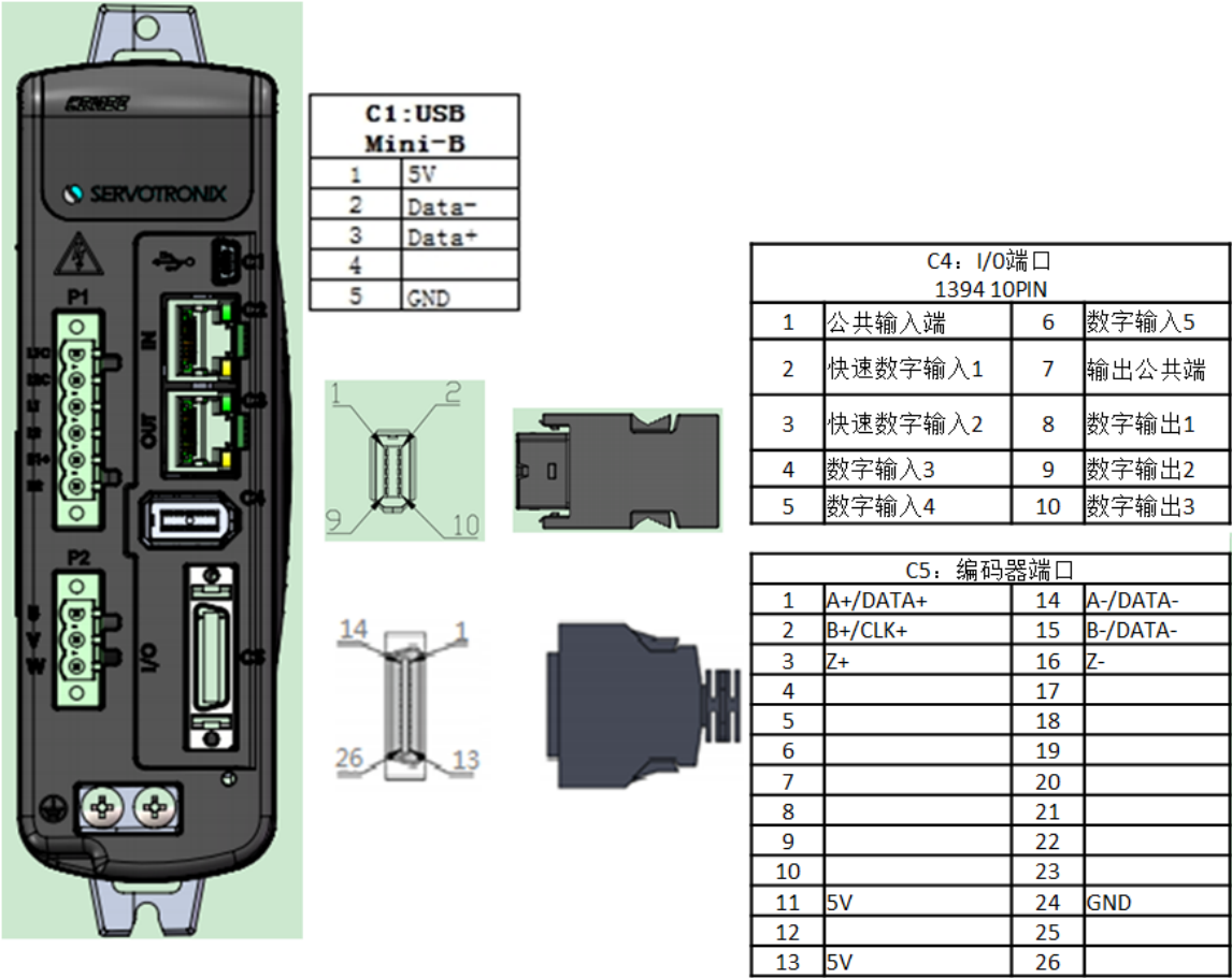
图 4-6 CDHDE-4D52AEB 控制板引脚分配
