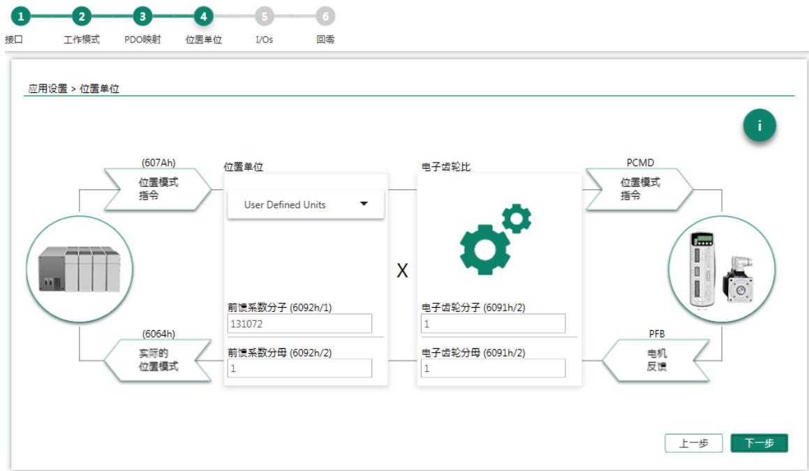
图 6 - 6-4. ServoStudio 2 - 应用程序设置向导 - 位置单位
