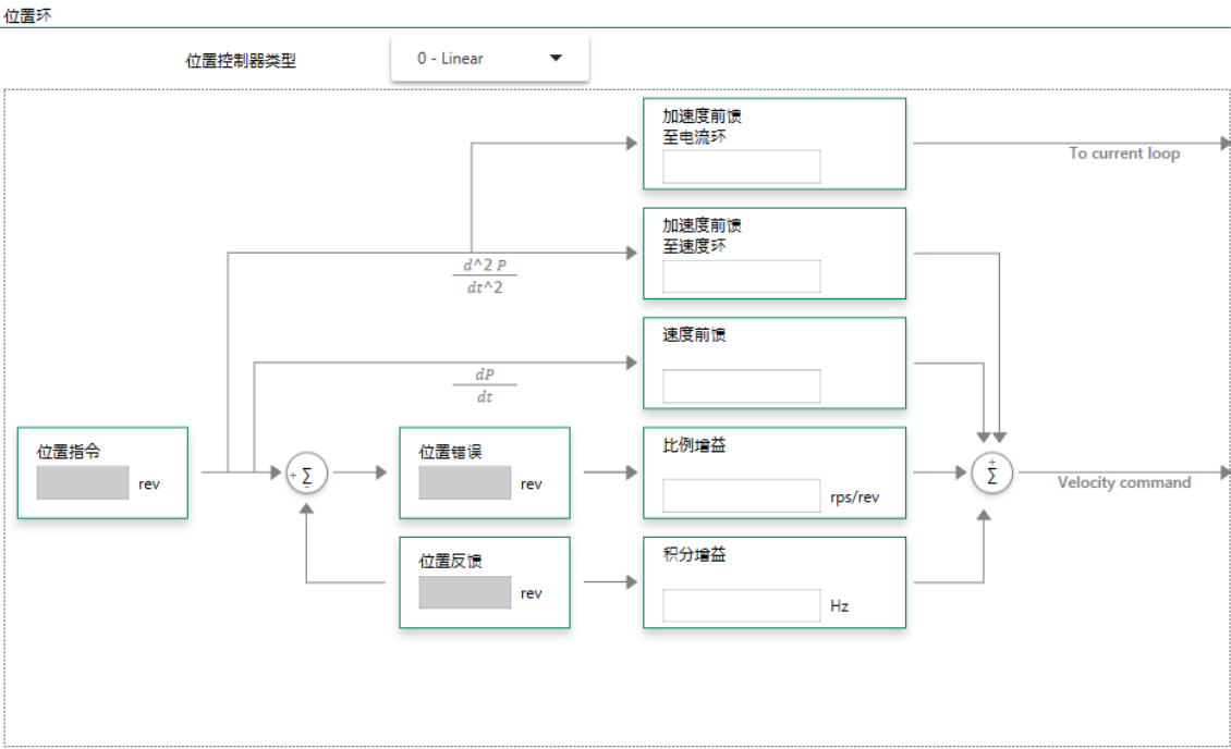
图 7 - 7-2. 位置控制环路 – 线性
