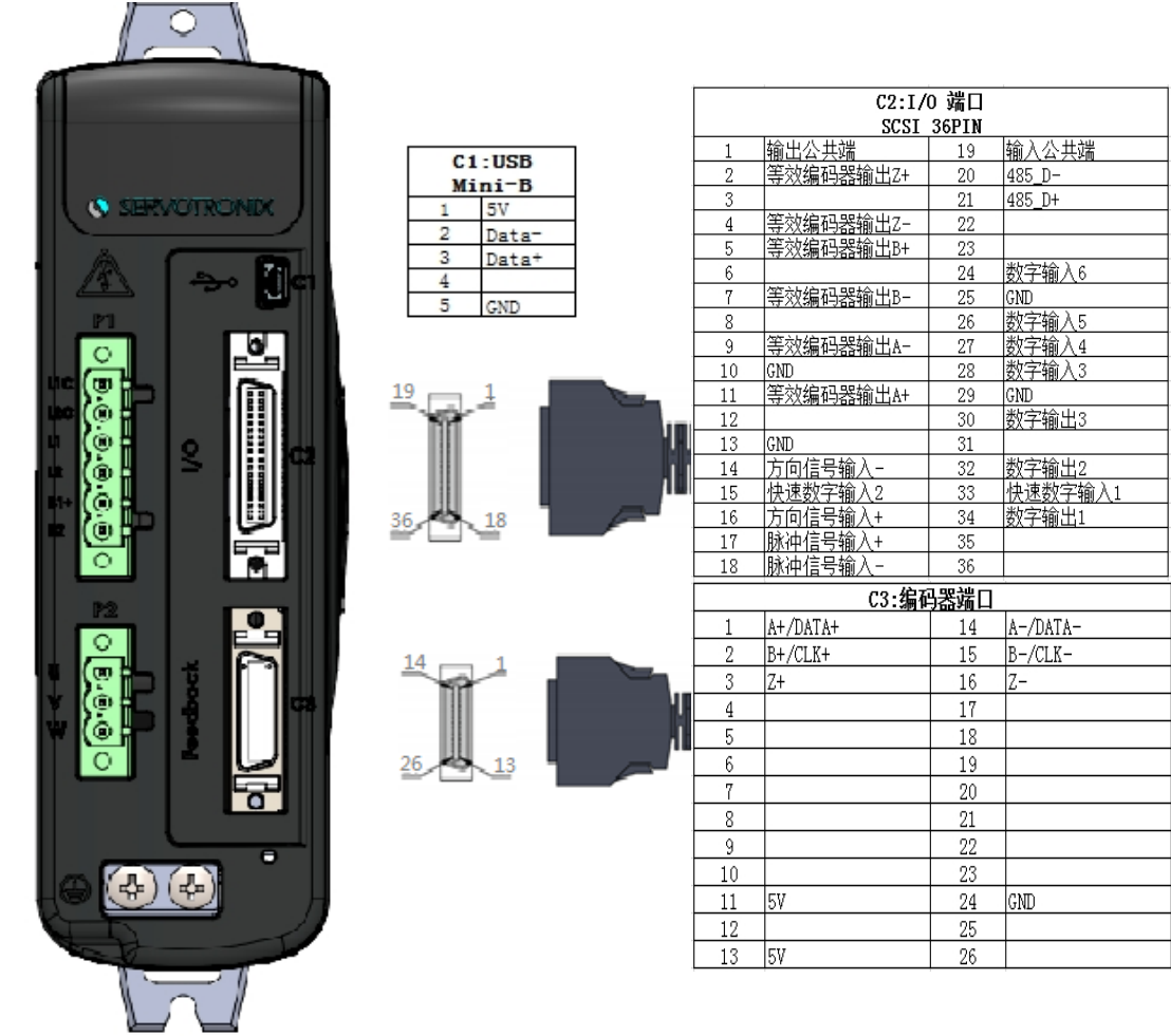
图 4-10 CDHDE-4D52AAP 控制板引脚分配
