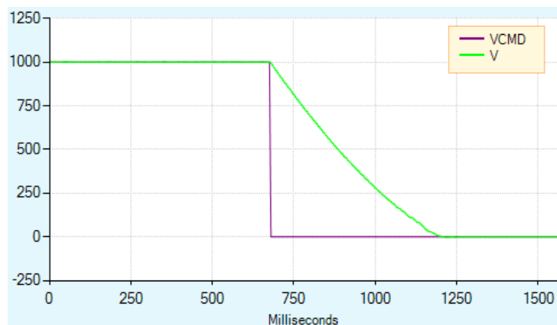
图 6 - 6-12. 在没有动态制动机制下电机滑行曲线
