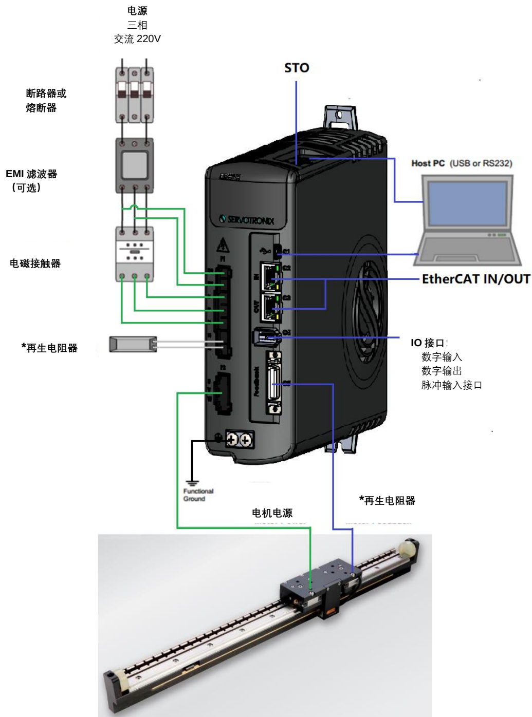
图 4-4 CDHDE-0102AEB 伺服系统接线
