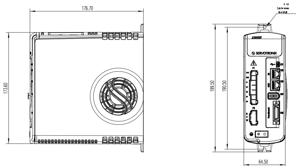
图 3-4 CDHDE-0102AEB 尺寸 (mm)
