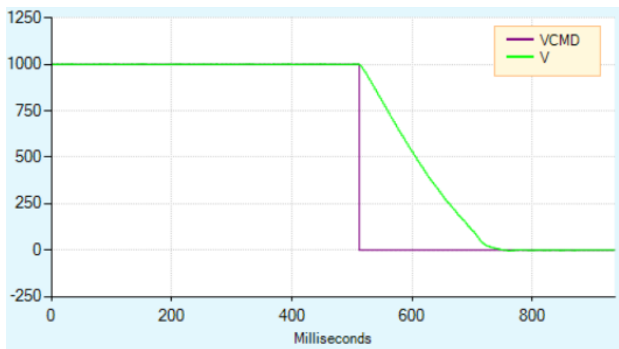
图 6 - 6-14. 在 ISTOP 值很小时动态制动曲线
