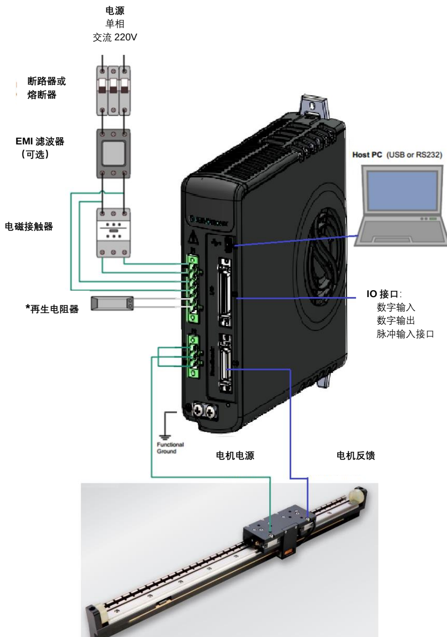
图 4 - 4-1. CDHDE-4D52AAP 伺服系统接线
