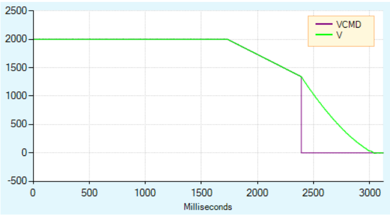
图 6 - 6-10. 第二禁用命令对活跃禁用的影响
