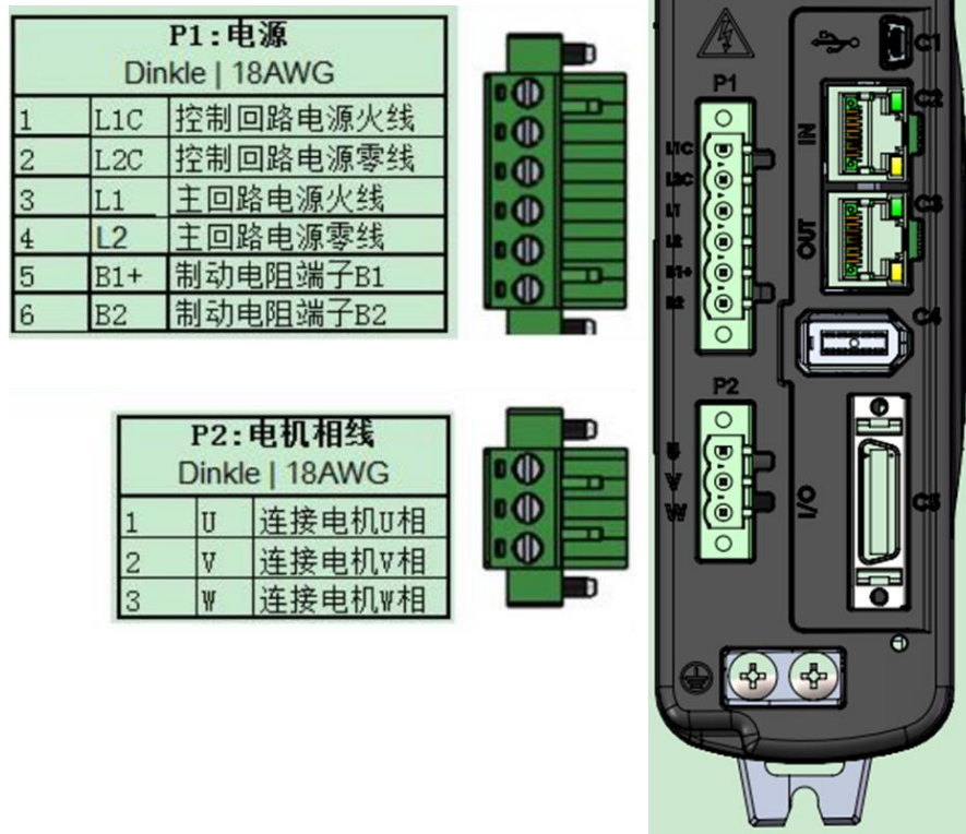
图 4 - 10. CDHDE-EB 电源板引脚分配
