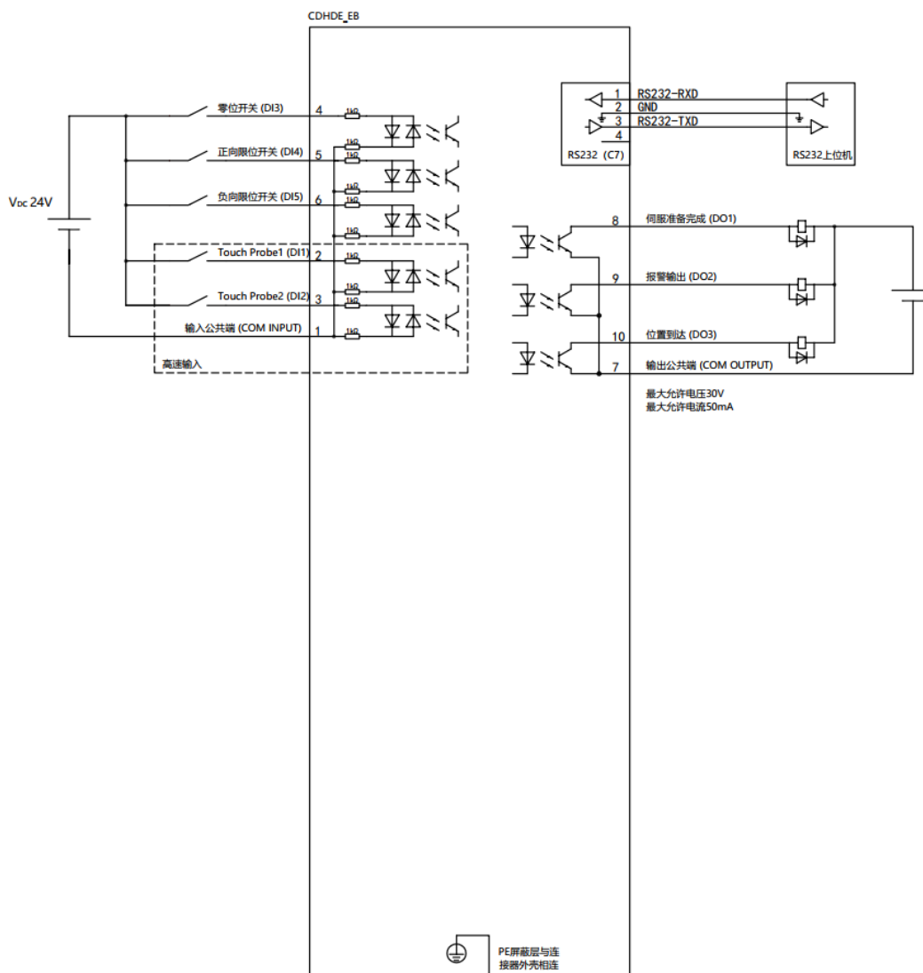
图 4-7 CDHDE-4D52AEB 默认 IO 接线图
