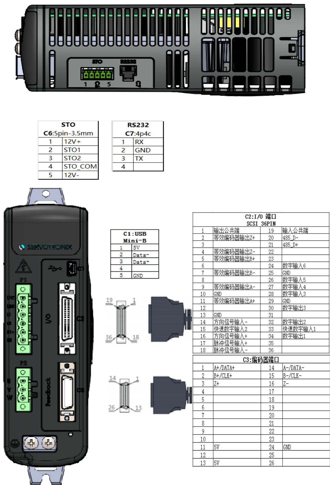
图 4 - 7. CDHDE-0102AAP 控制板引脚分配
