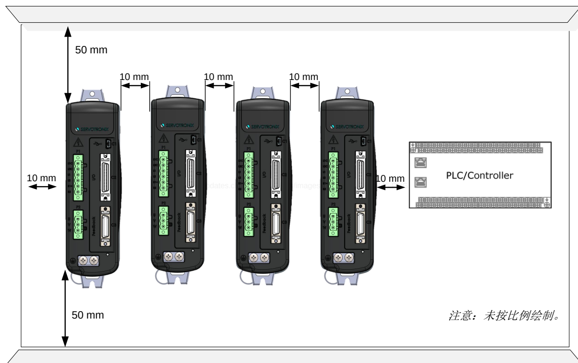
图 4 - 4-5. 在机柜内安装多个 CDHDE 单元
