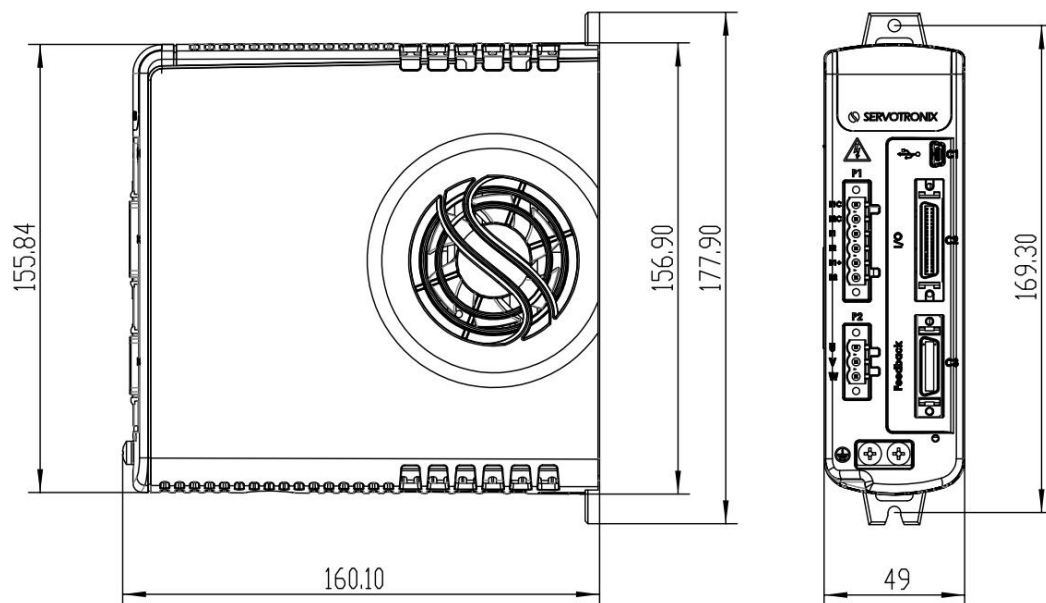
图 3-1. CDHDE-4D52AAP 尺寸 (mm)
