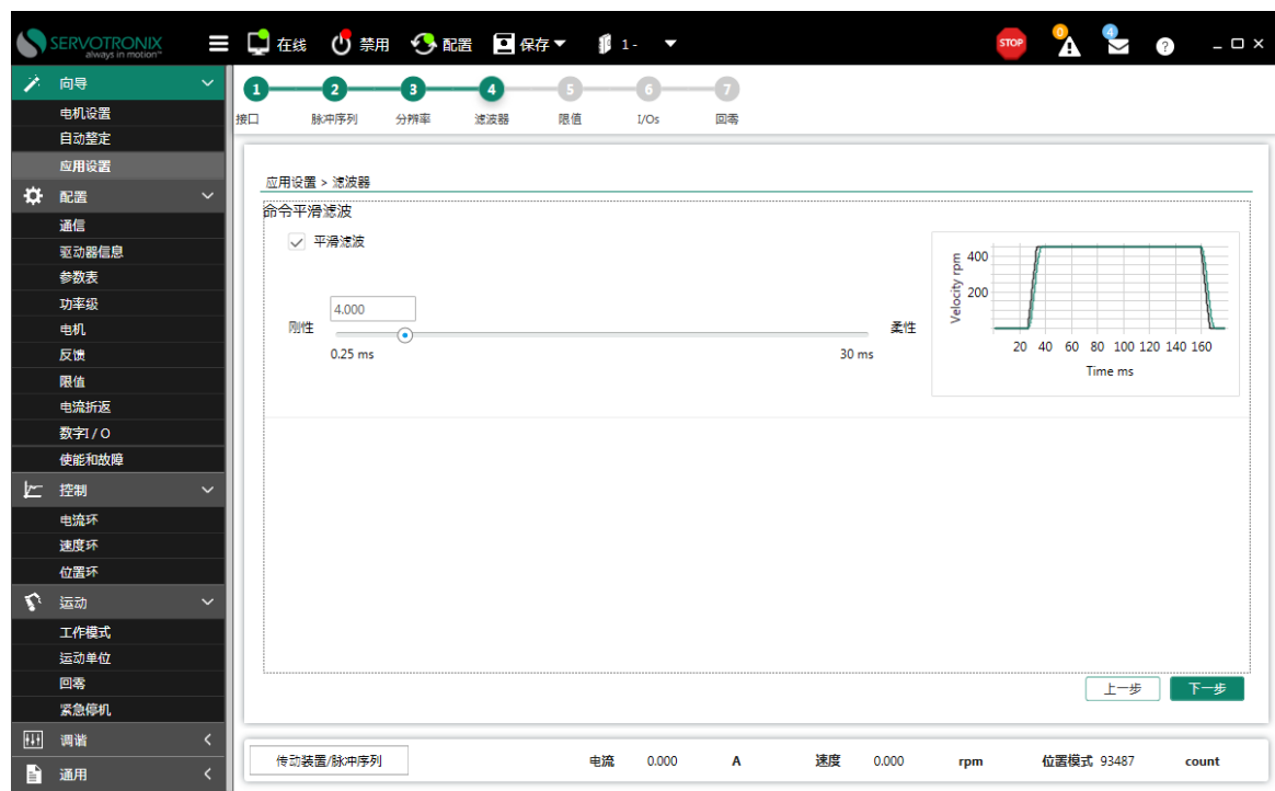
图 7 - 7-6. ServoStudio 2 - 应用程序设置向导 - 滤波器
