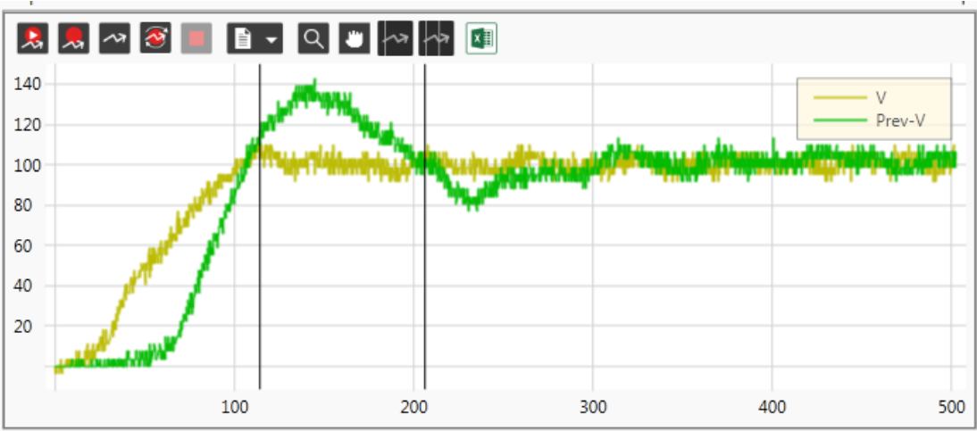
图 8 - 8-1. 依据辨识结果设置质量比前后速度响应曲线
