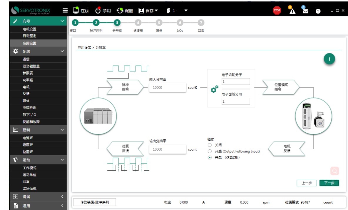
图 7 - 7-5. ServoStudio 2 - 应用程序设置向导 - 分辨率
