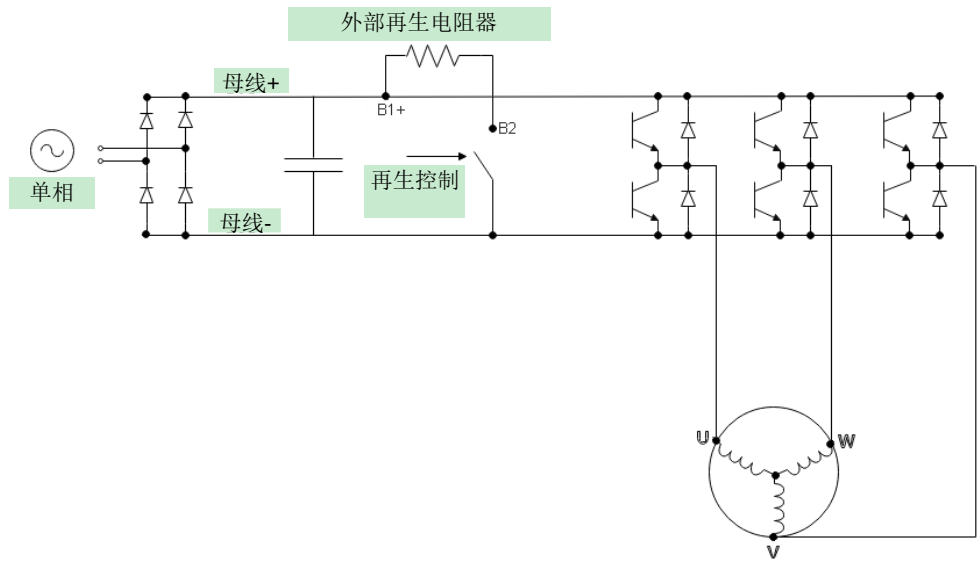
图 4 - 12. 再生电阻器电路
