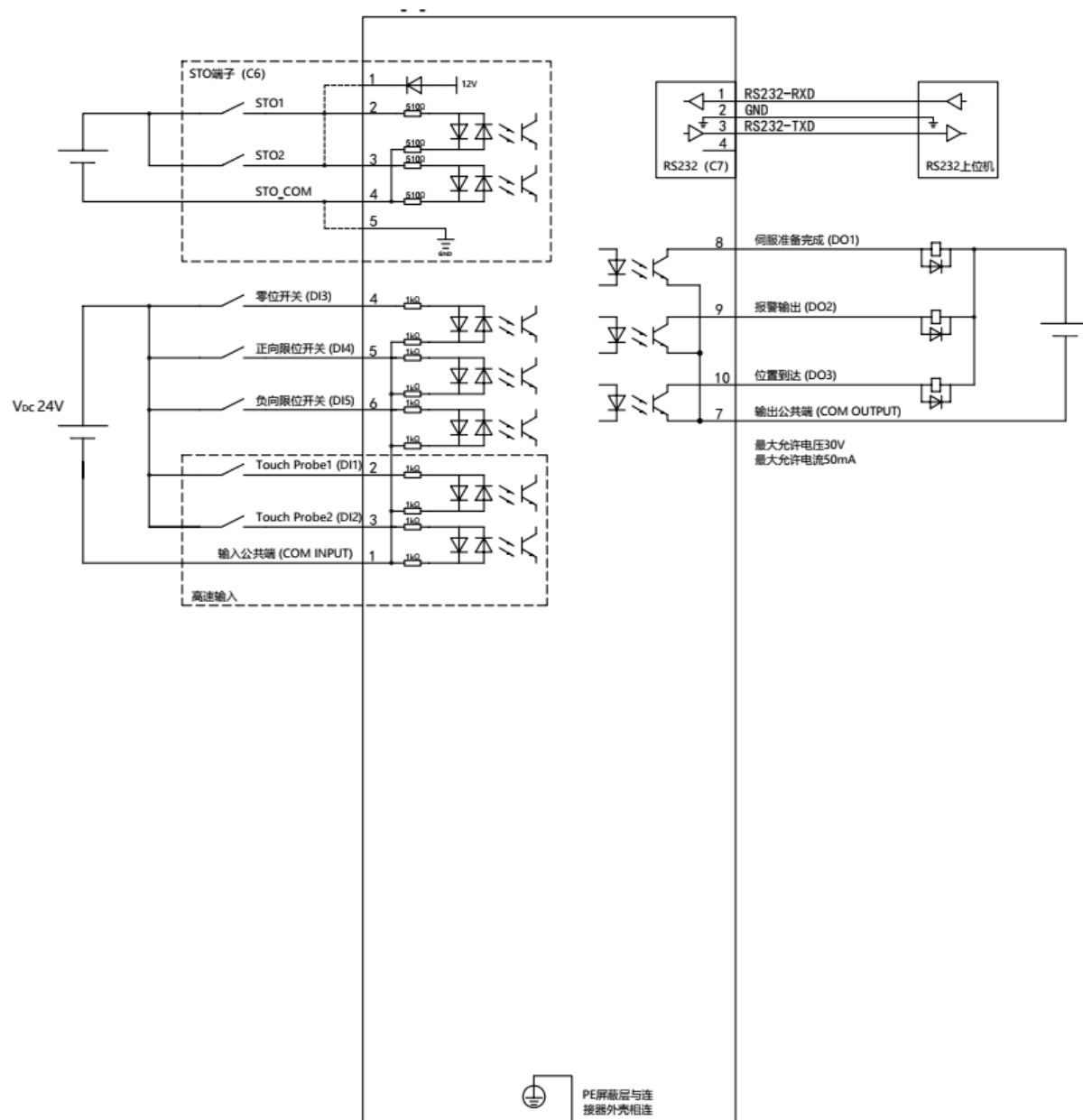
图 4-9 CDHDE-0102AEB 默认 IO 接线图
