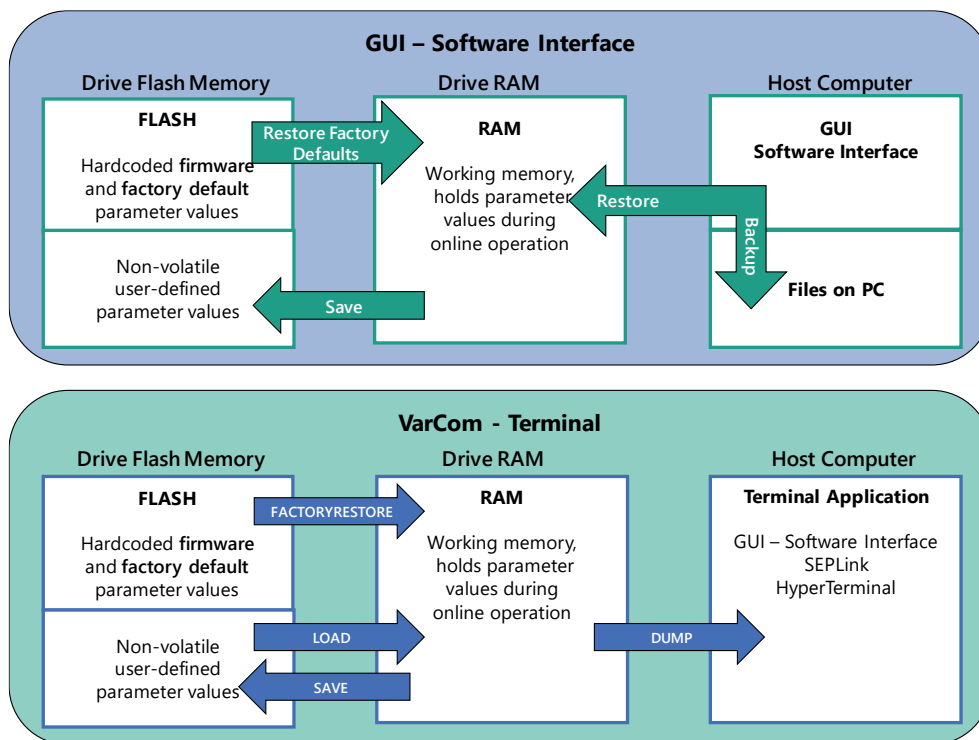
图 6 - 6-1. 存储器与参数管理命令
