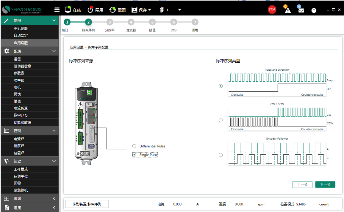
图 7 - 7-4. ServoStudio 2 - 应用程序设置向导 - 脉冲序列配置
