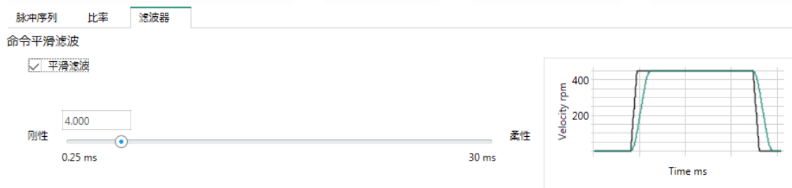
图 7 - 7-14. ServoStudio 2 - 运动 - 操作模式 - 脉冲序列 - 滤波器
