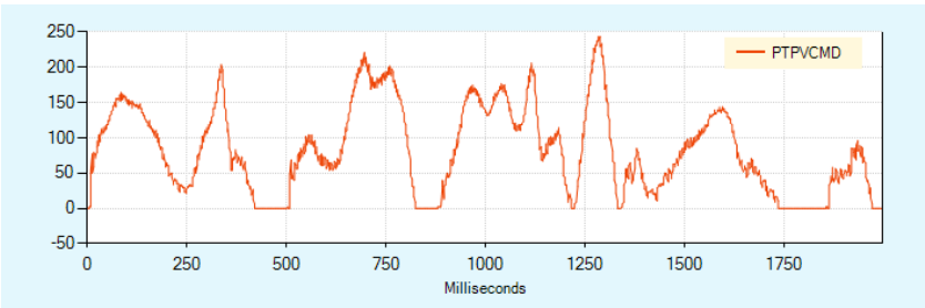
图 8 - 8-5. PTPVCMD 效果不佳
