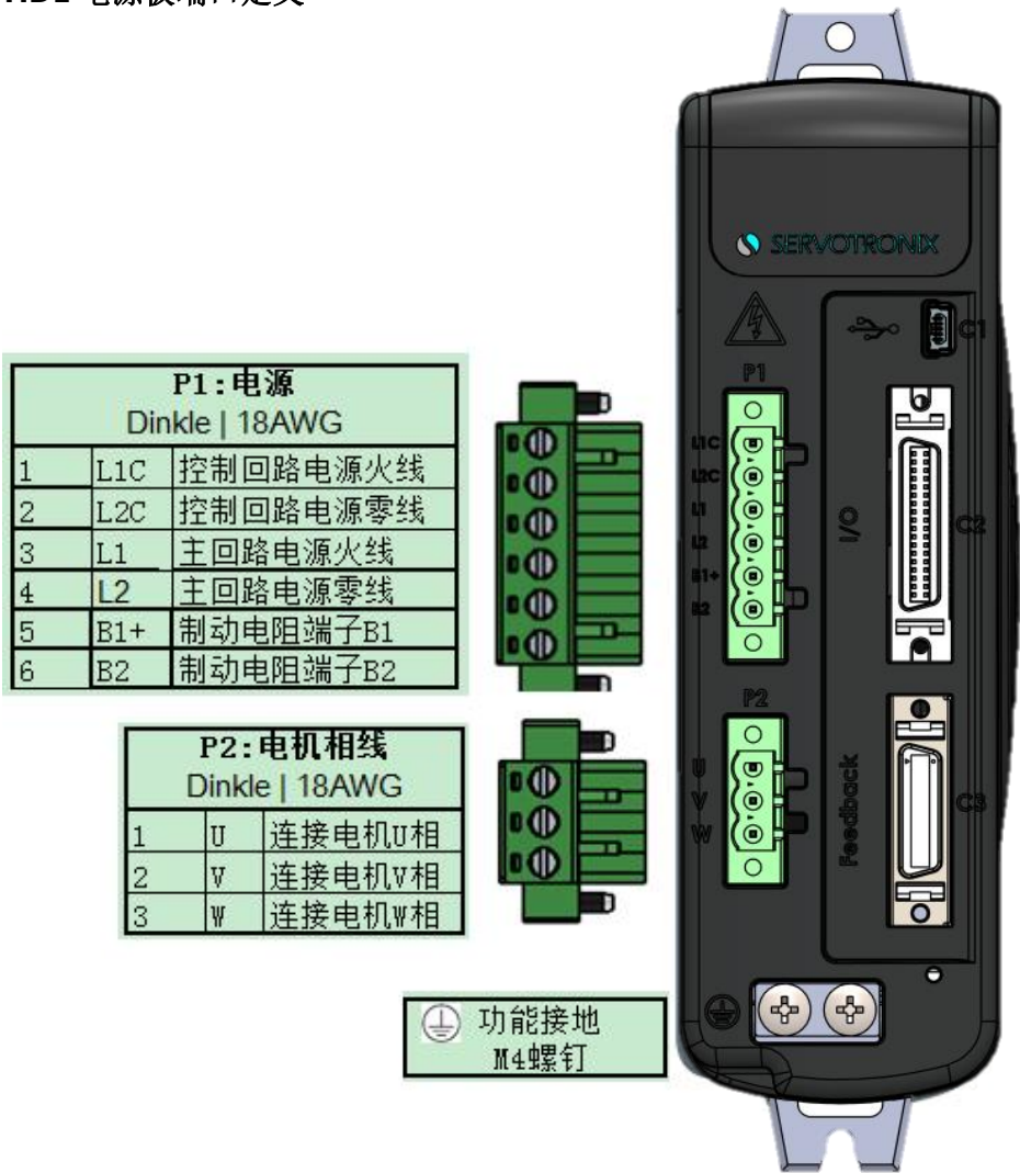
图 4 - 9. CDHDE-AP 电源板引脚分配
