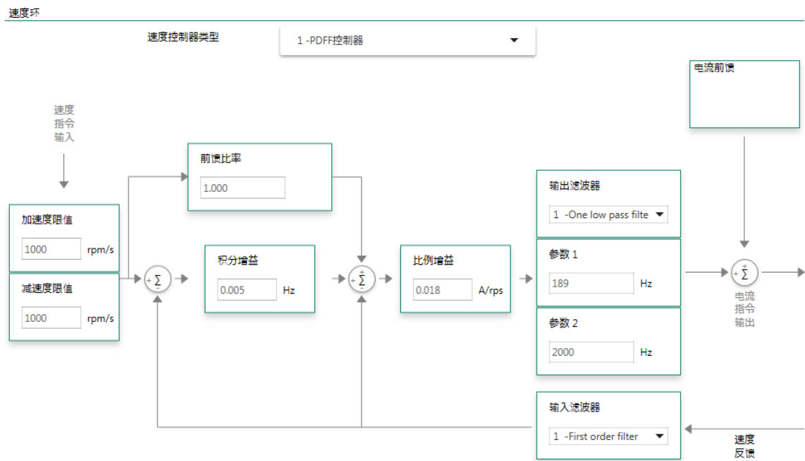
图 7-7-1. 速度控制回路 – PDFF 控制器
