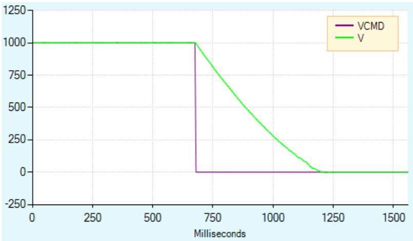
图 6 - 6-7. 禁用（不使用活跃禁用）
