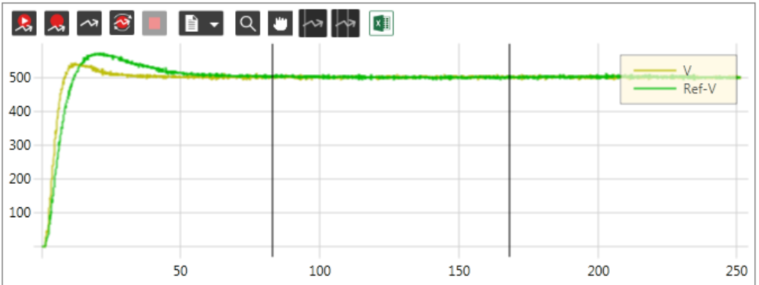
图 8 - 8-2. 不同刚性的速度响应（1）
