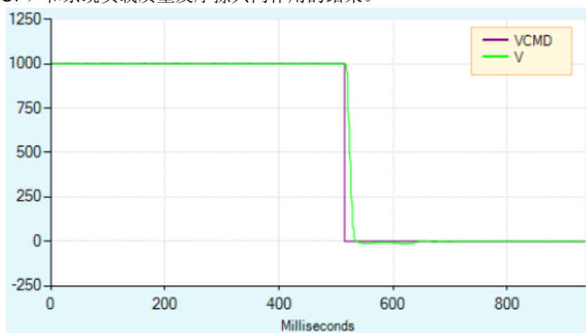
图 6 - 6-13. 动态制动曲线
