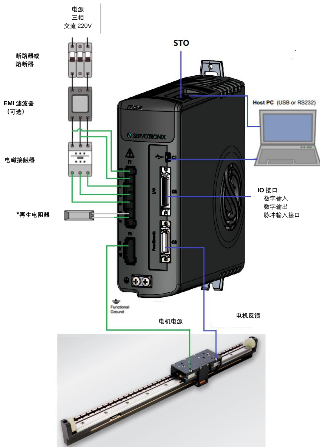
图 4-3 CDHDE-0102AAP 伺服系统接线
