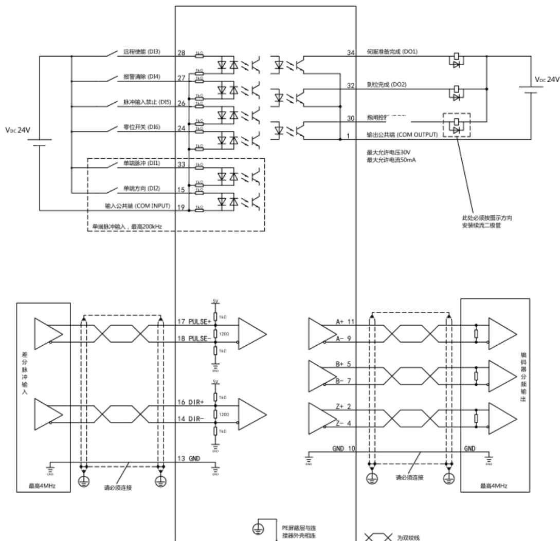
图 4-11 CDHDE-4D52AAP 默认 IO 接线图
