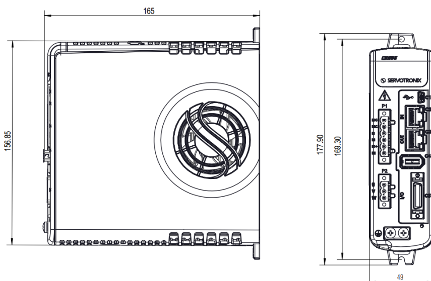
图 3-2 CDHDE-4D52AEB 尺寸 (mm)
