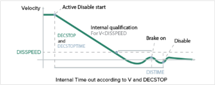
图 6 - 6-11. 禁用停止
