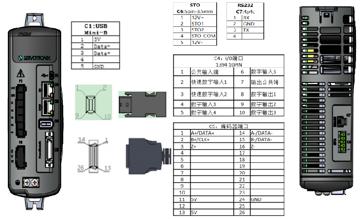
图 4-8 CDHDE-0102AEB 控制板引脚分配
