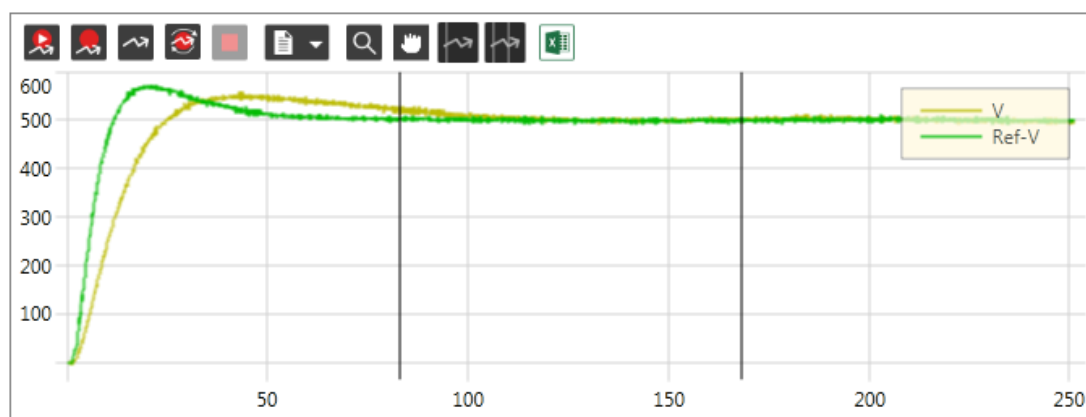
图 8 - 8-3. 不同刚性的速度响应 (2)
