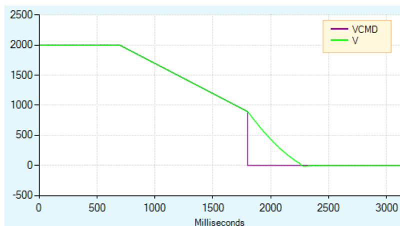
图 6 - 6-9. DISSPEED 和 DISTIME 对活跃禁用的影响
