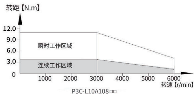
转矩特性图
