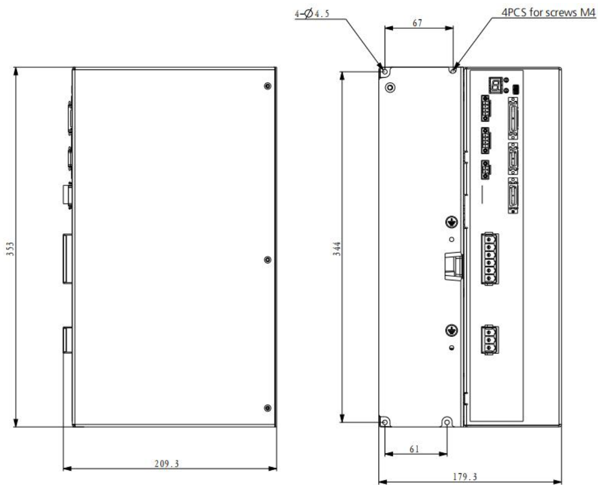
图 3-6 CDHD2S-040(高压) - 尺寸(mm)
