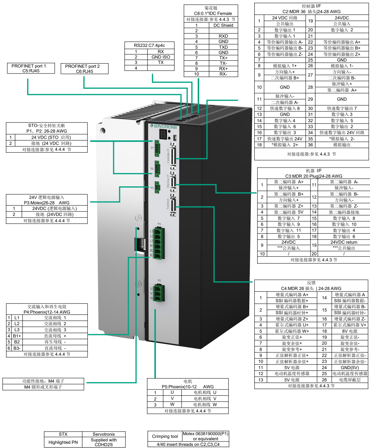
图 4-33 CDHD2S-040(高压 PN-R0 型号)功率板引脚分配
