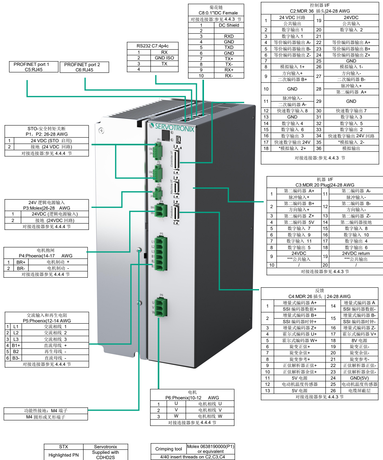
图 4-32 CDHD2S-024/CDHD2S-030 (高压 PN-R0 型号) 功率板引脚分配
