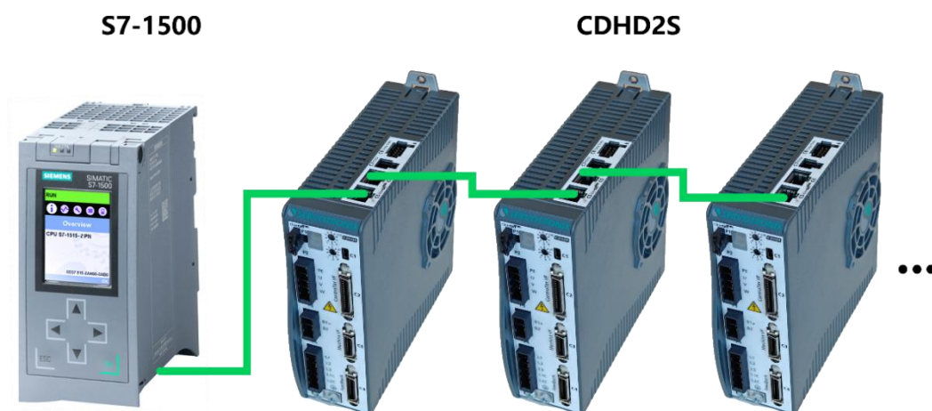
图 9-2 SERVOTRONIX CDHD2S-PN 与 Siemens S7-1500 硬件拓扑
