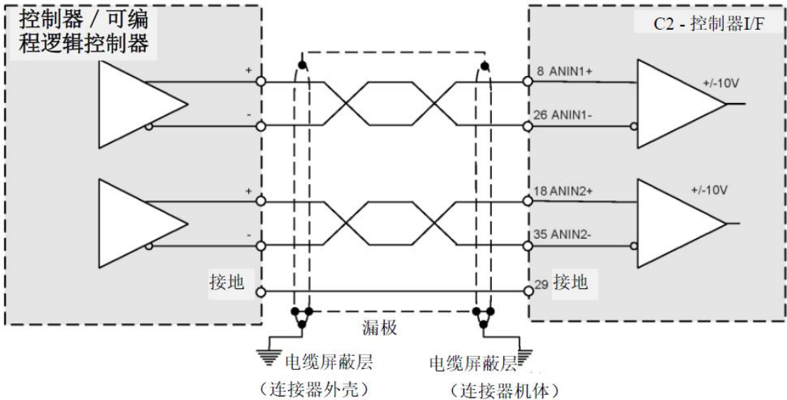
图 4-18 模拟输入接线-C2
