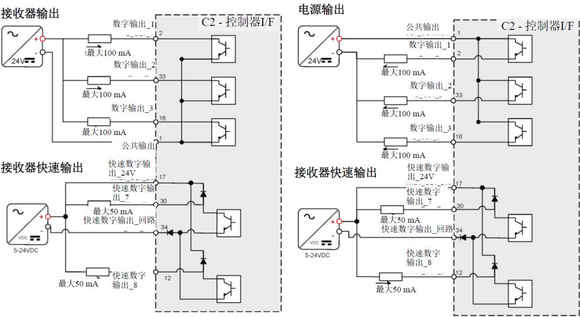
图 4-17 数字输出接线 - C2
