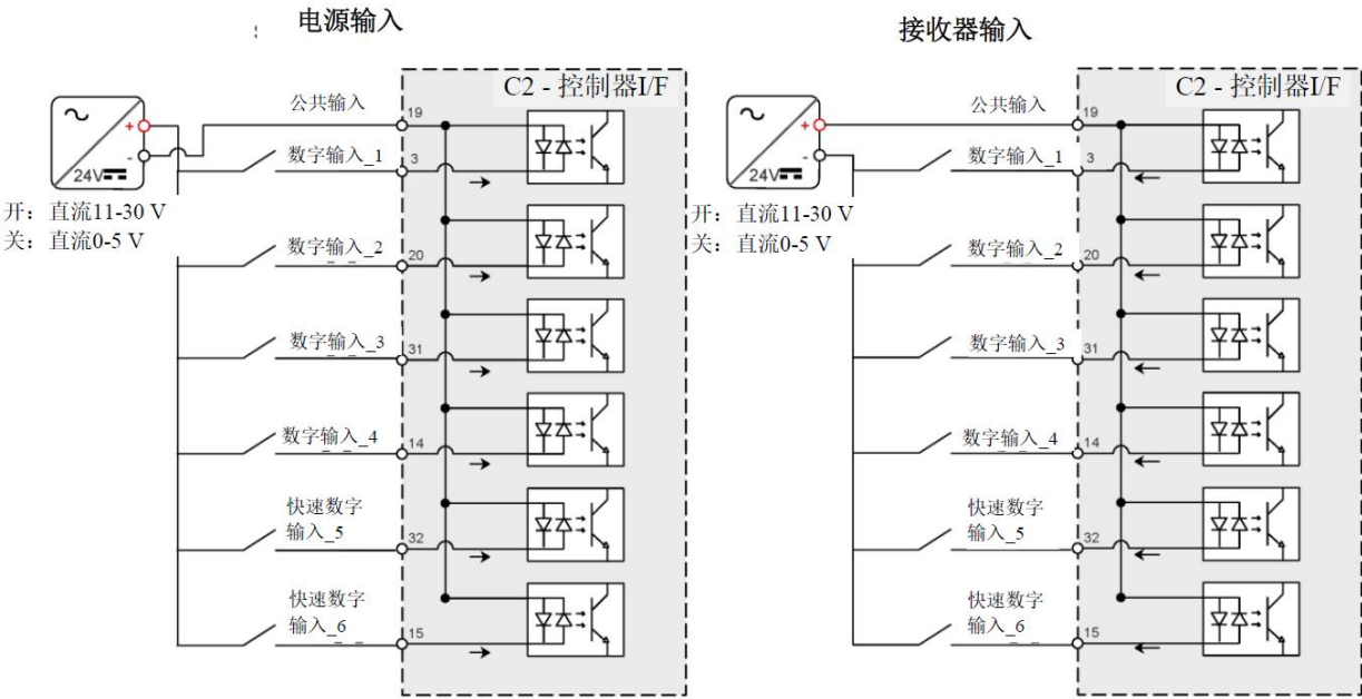
图 4-16 数字输入接线-C2
