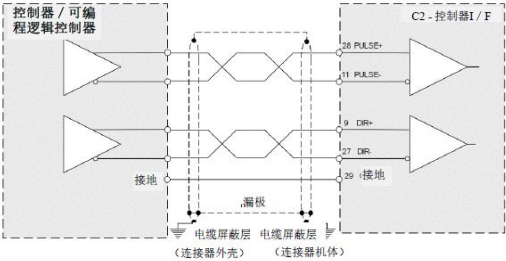
图 4-21 脉冲和方向光学隔离输入接线 - C2
