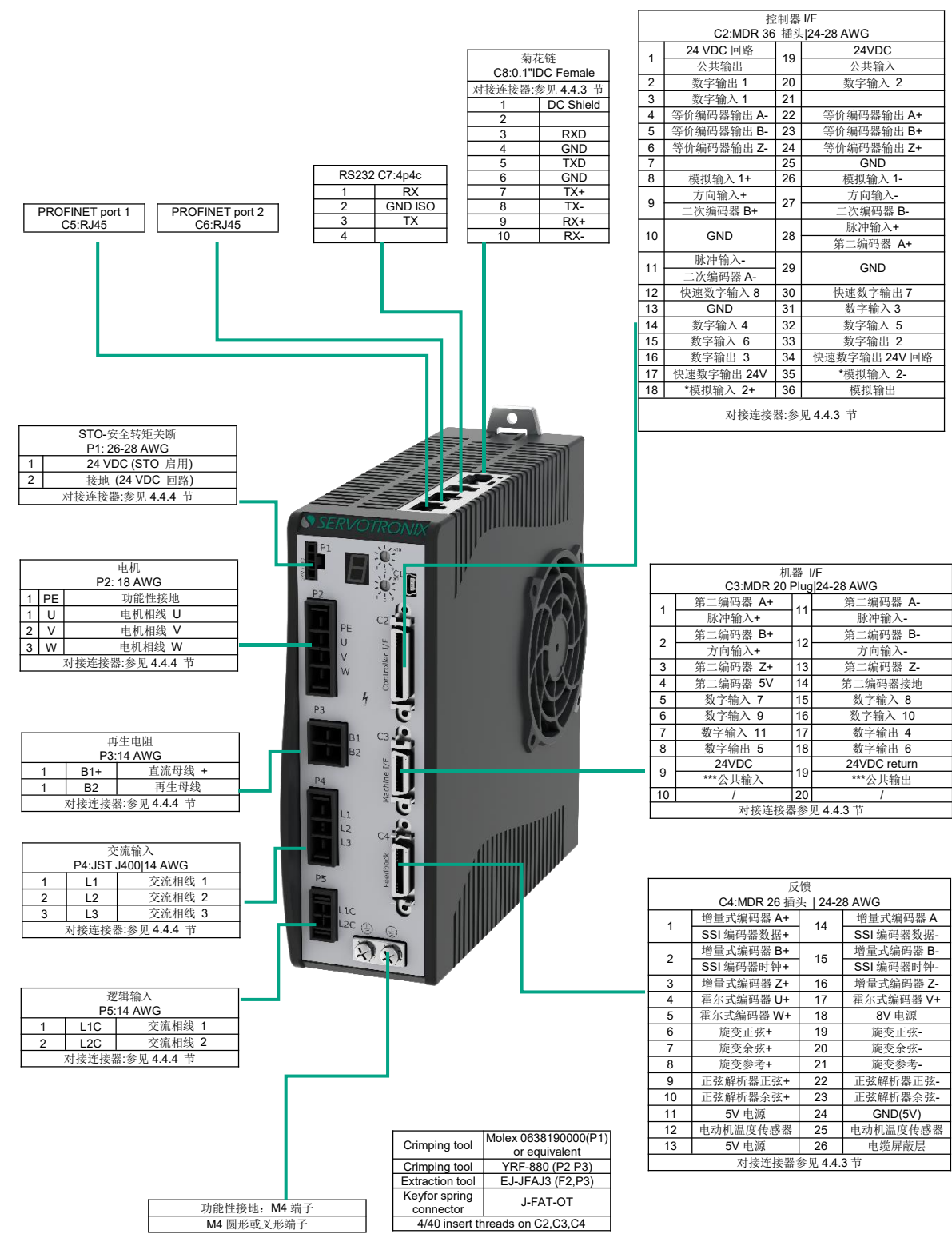
图 4-30 CDHD2S-010(中压 PN-R0 型号)功率板引脚分配
