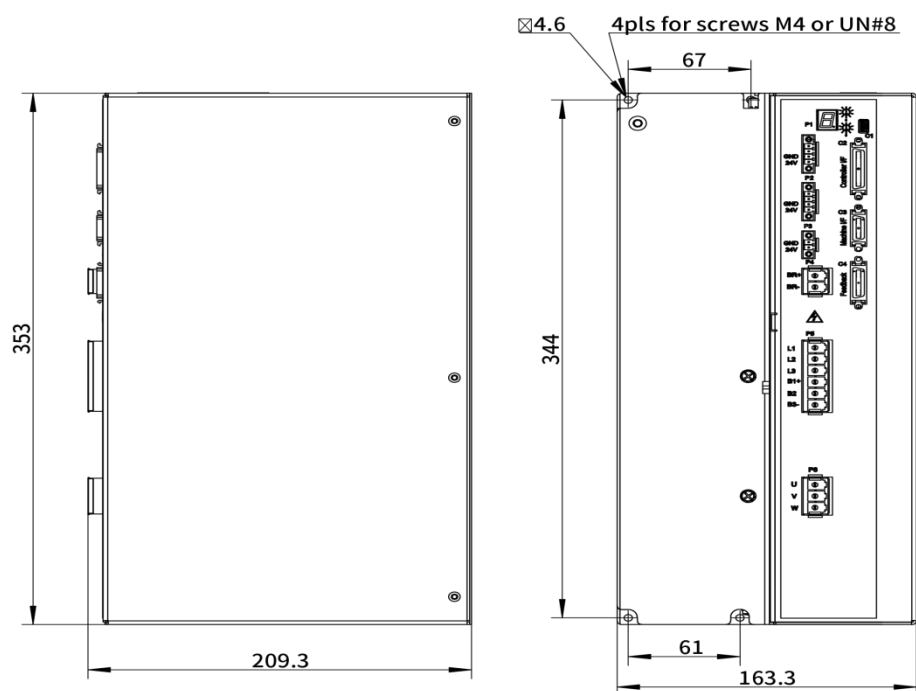
图 3-5 CDHD2S-024/CDHD2S-030(高压) - 尺寸(mm)
