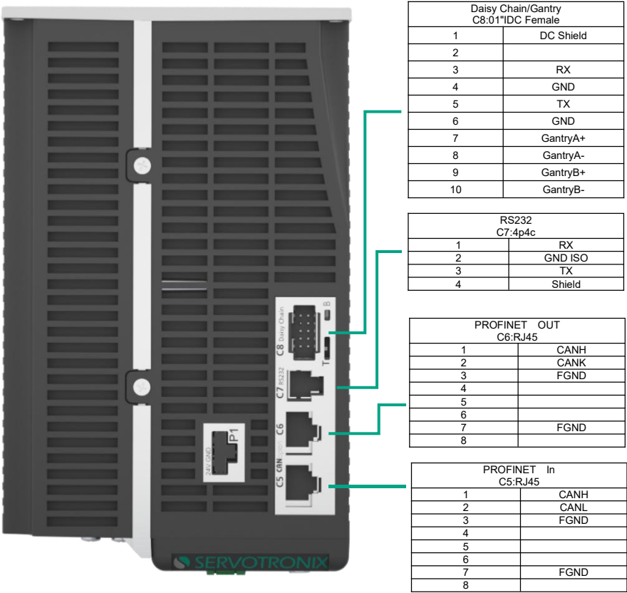
图 4-15 CDHD2S PN-R0 型号上面板引脚分配
