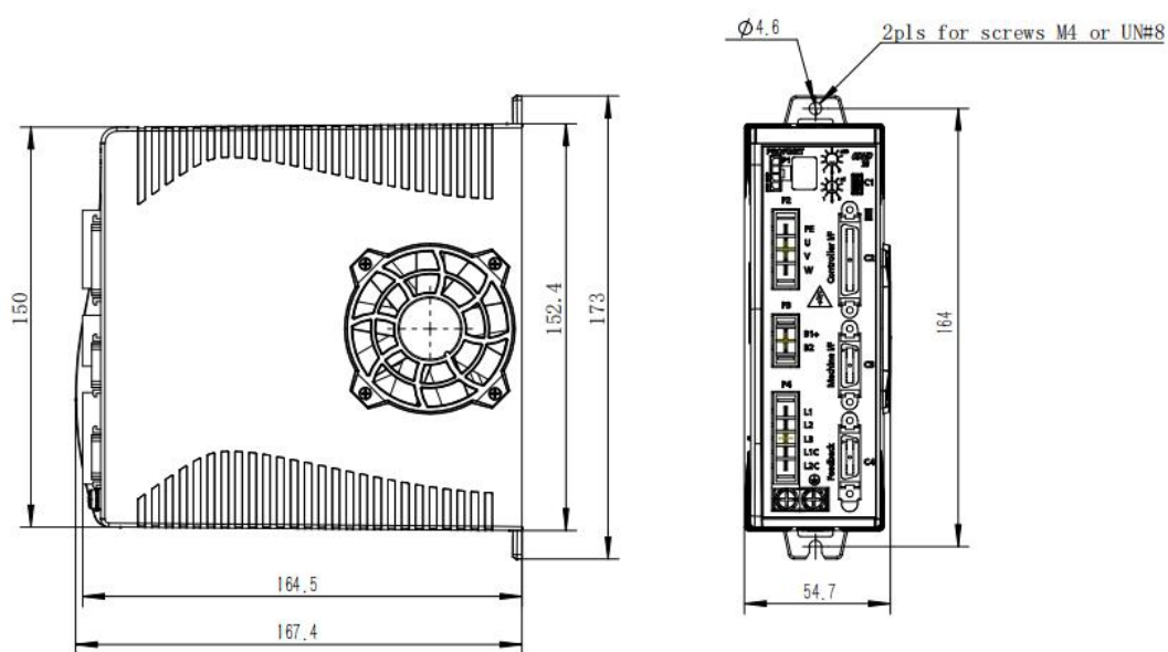
图 3-2 CDHD2S-006(中压 PN 机型) - 尺寸(mm)
