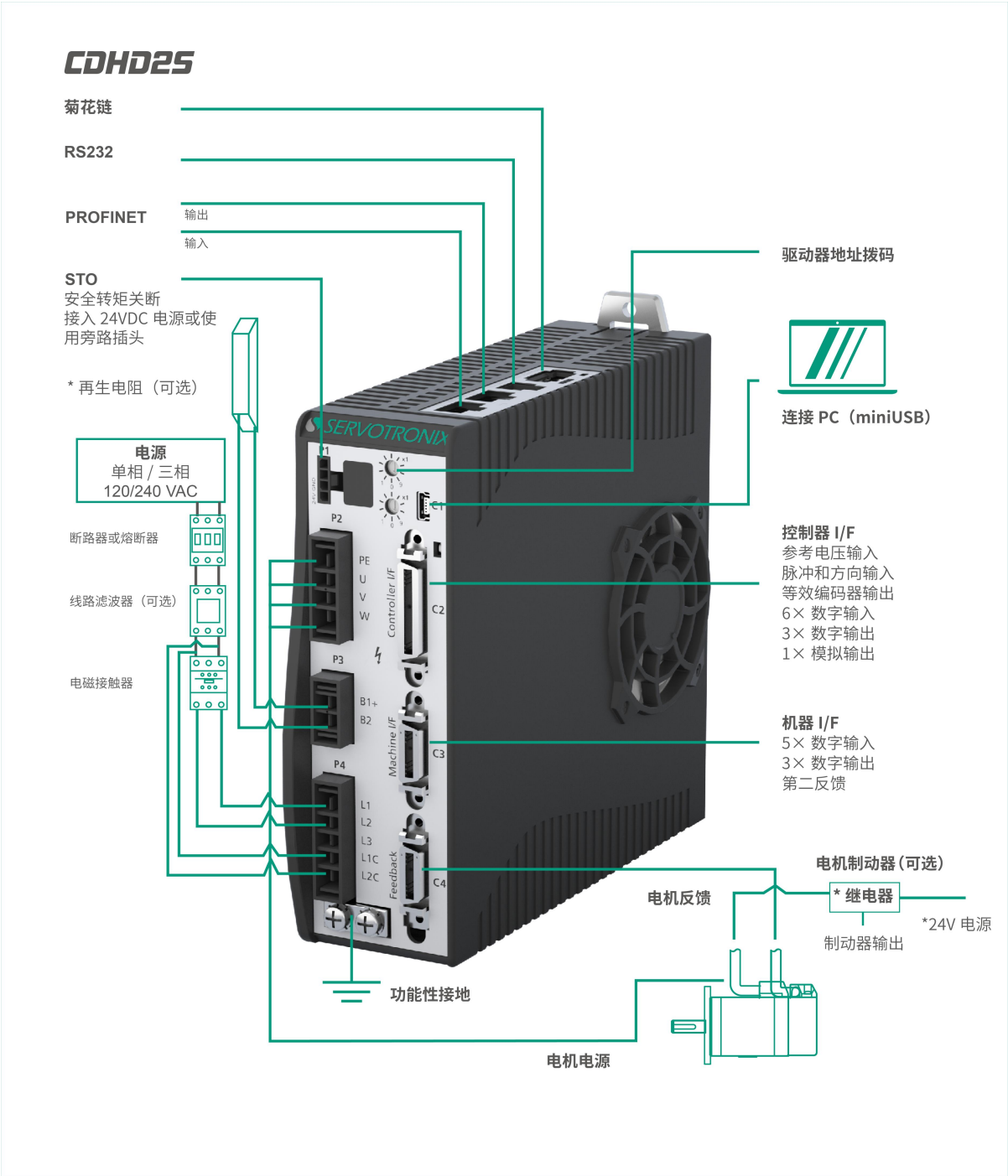
图 4-4 CDHD2S-006 交流 120-240V (中压 PN-R0) 型号系统接线
