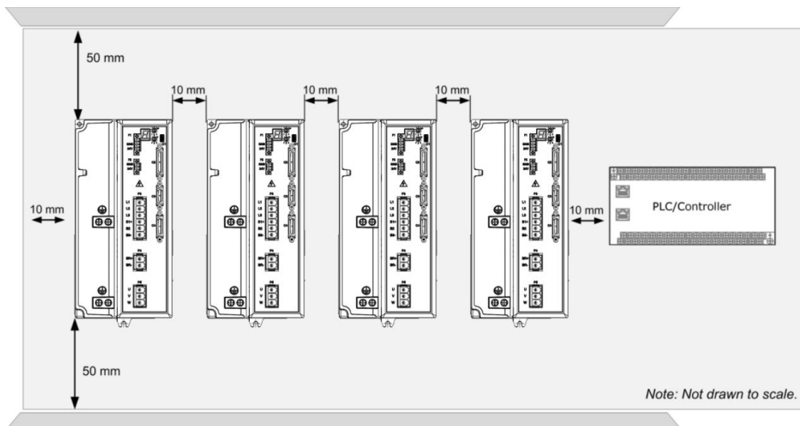
图 4-12 在机柜内安装多个 CDHD2S 单元
