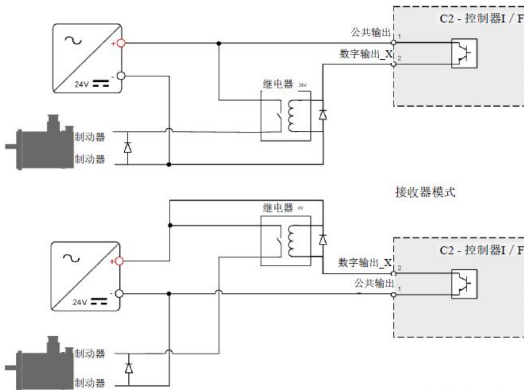
图 4-25 电机制动器接线 CDHD2S (中压型号)
