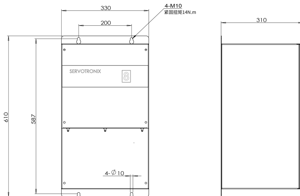
图 3-7 CDHD2S-060(高压) - 尺寸(mm)
