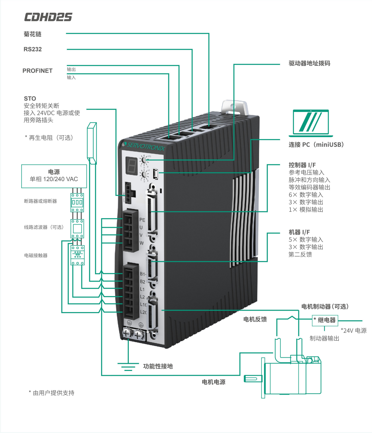
图 4-3 CDHD2S-003 交流 120-240V(中压 PN-R0)型号系统接线
