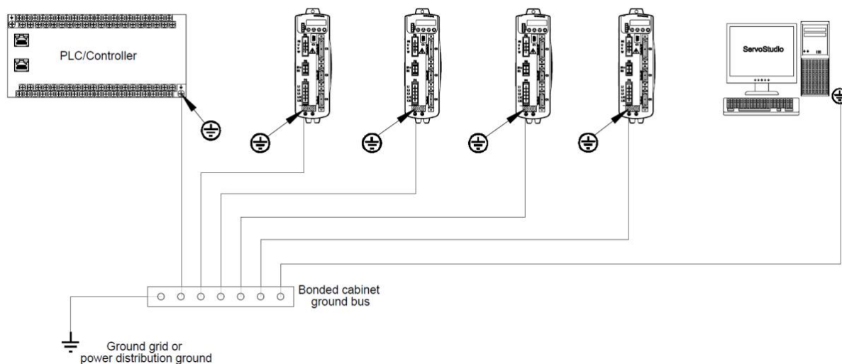
图 4-10 CDHD2S 系统接地
