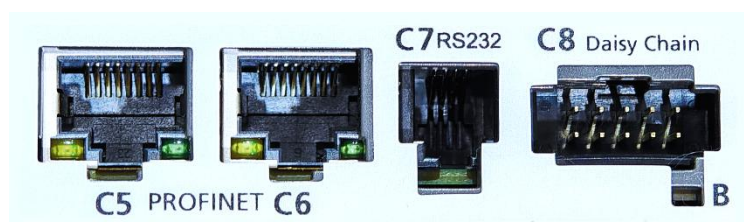
图 9-1 CDHD2S-PN 顶部面板的接口
