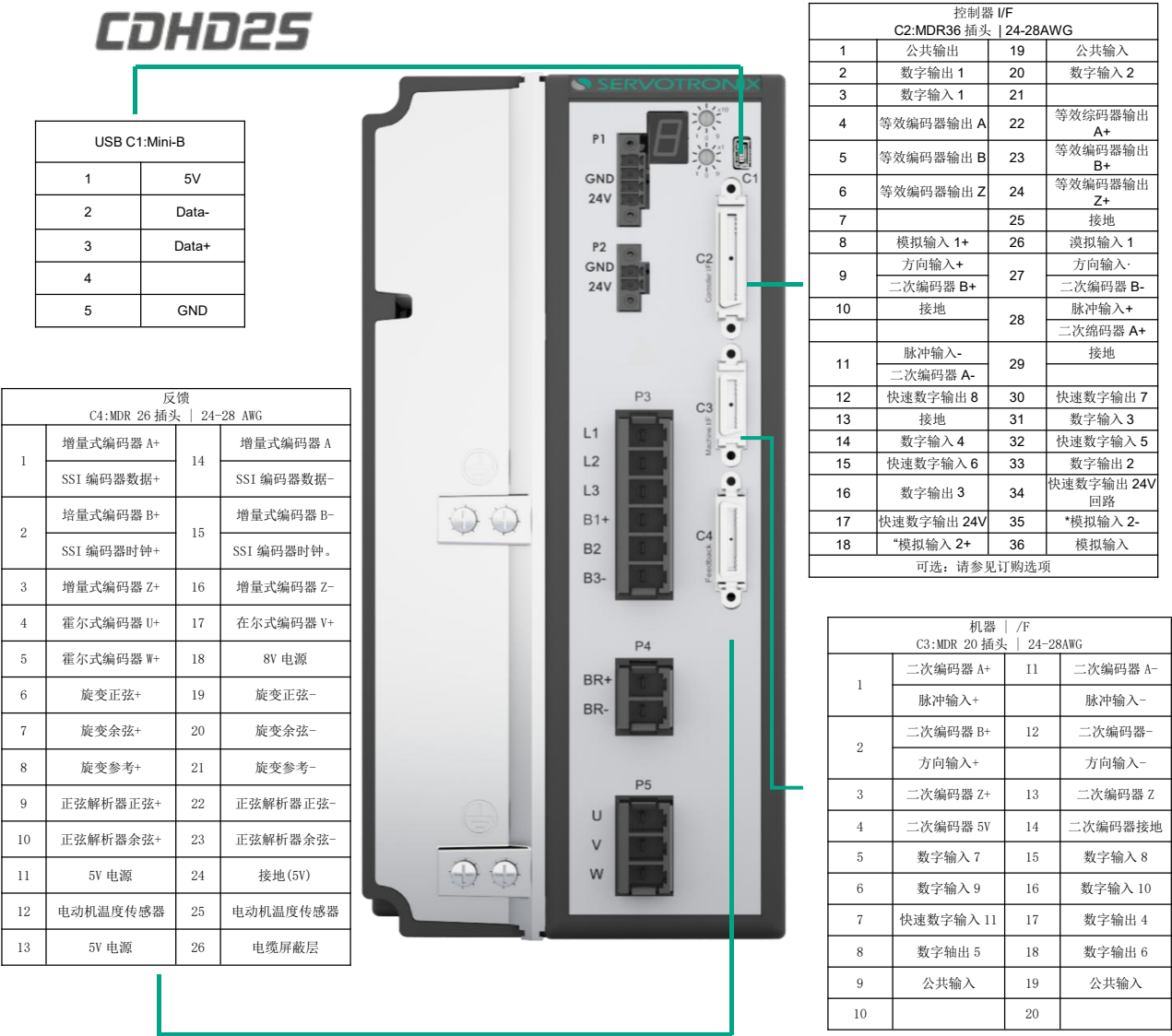
图 4-14 CDHD2S-12A/24A/30A/40A 高压 PN-RO 型号控制板引脚分配
