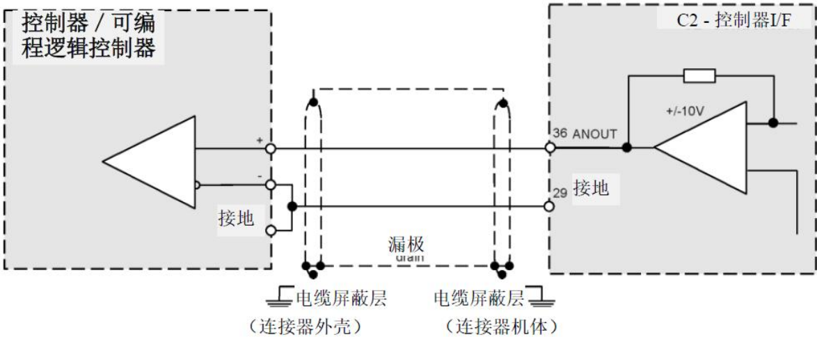
图 4-19 模拟输出接线 - C2
