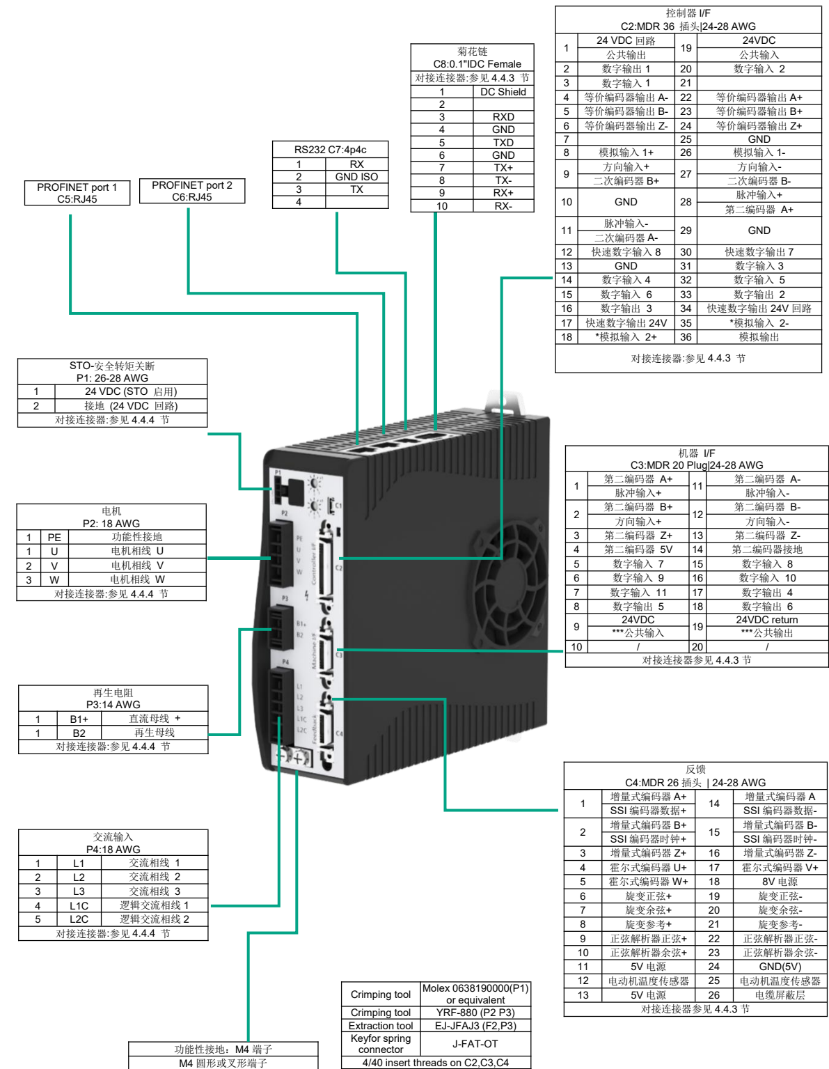
图 4-29 CDHD2S-006(中压 PN-R0 型号)功率板引脚分配
