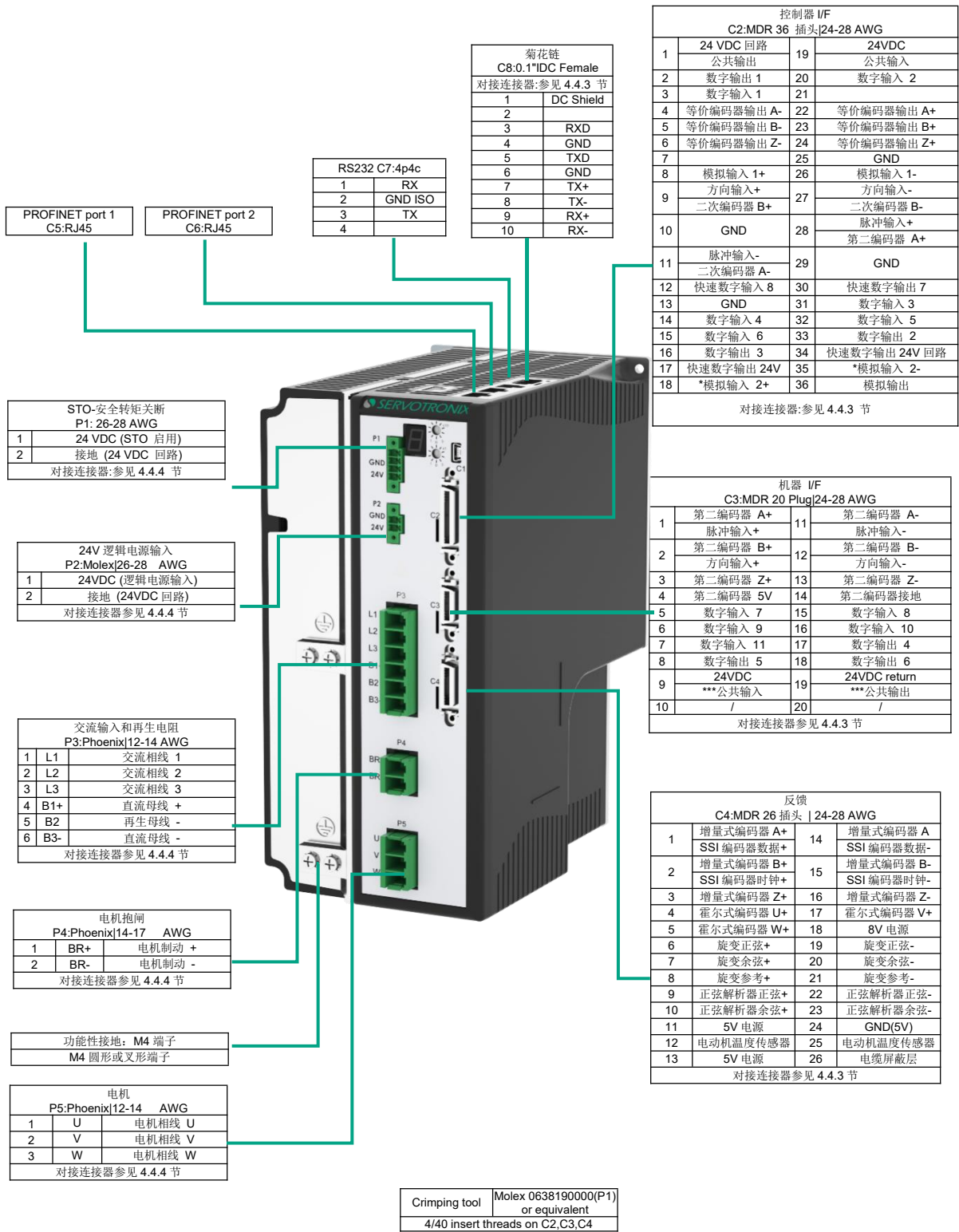
图 4-31 CDHD2S-012(高压 PN-R0 型号)功率板引脚分配
