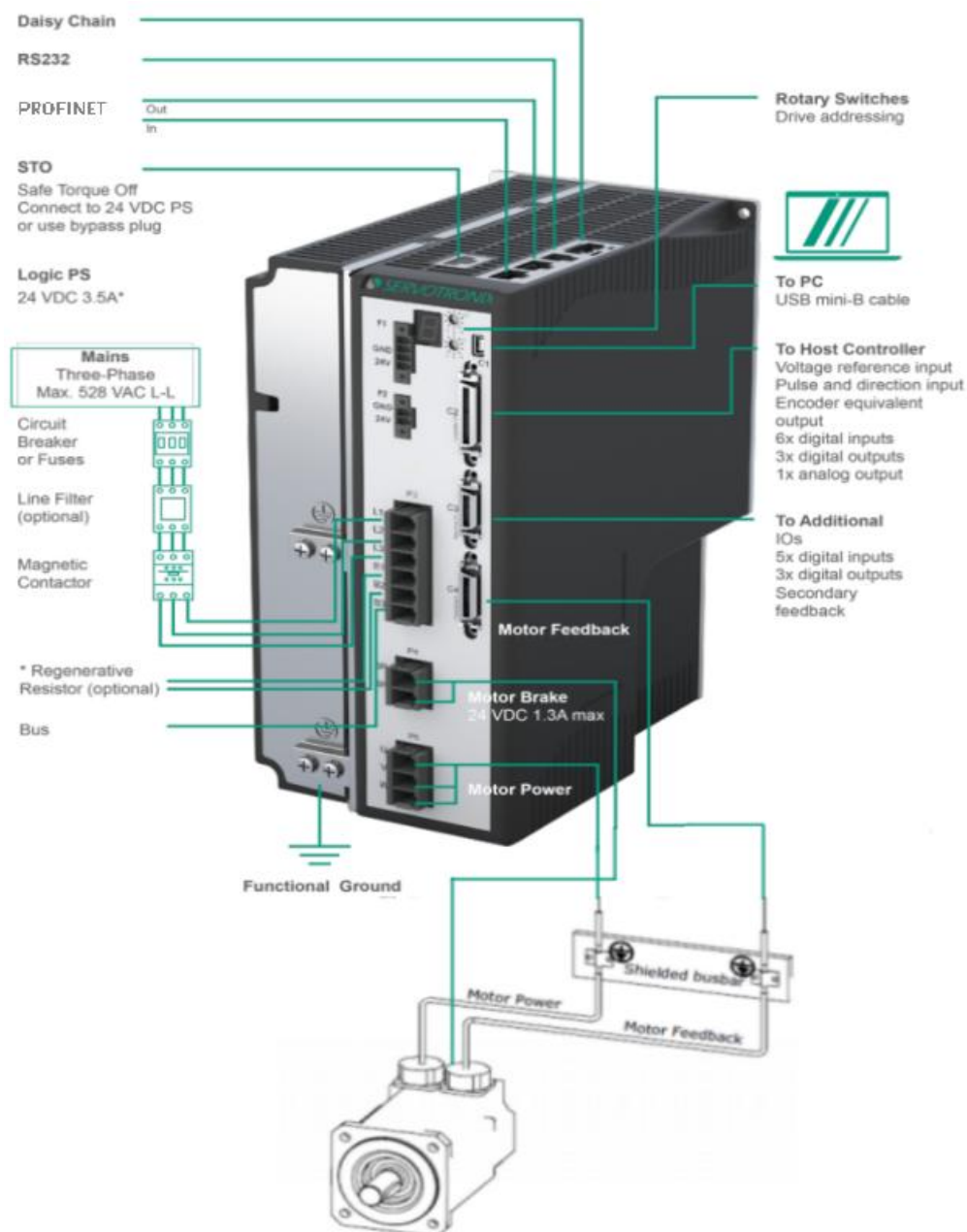
图 4-11 电机动力电缆和反馈电缆接地示意图
