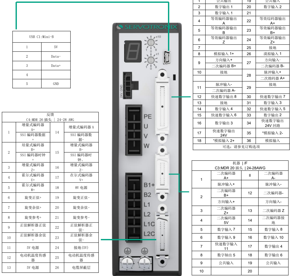
图 4-13 CDHD2S-3A/6A/10A 中压 PN-R0 型号控制板引脚分配
