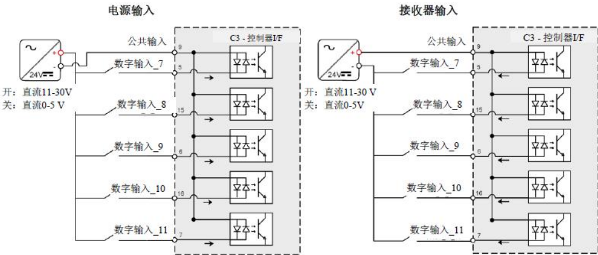
图 4-23 数字输入接线 - C3
