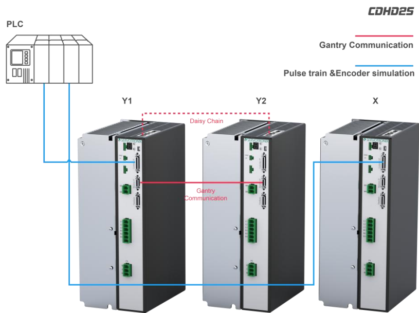
图 4-26 龙门系统接线 - 脉冲方向和串行
