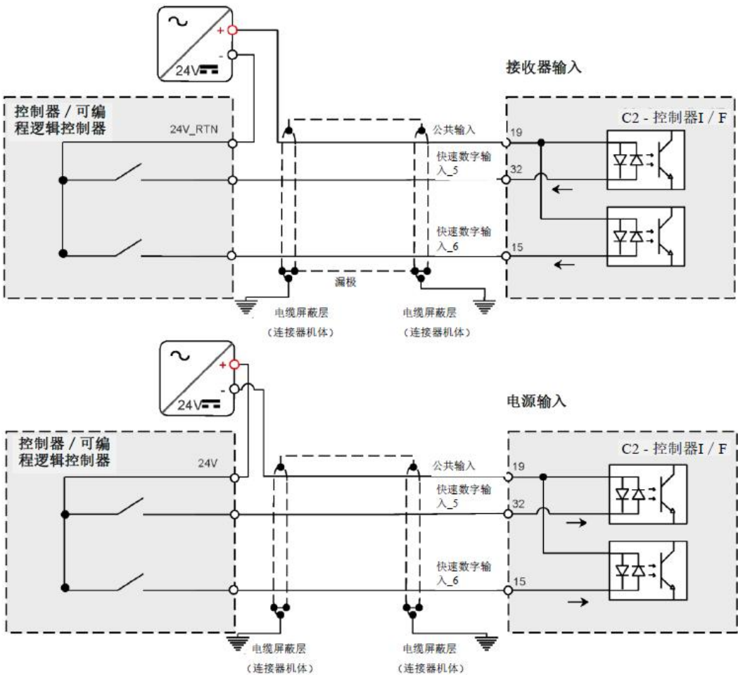
图 4-20 脉冲和方向光学隔离输入接线-C2
