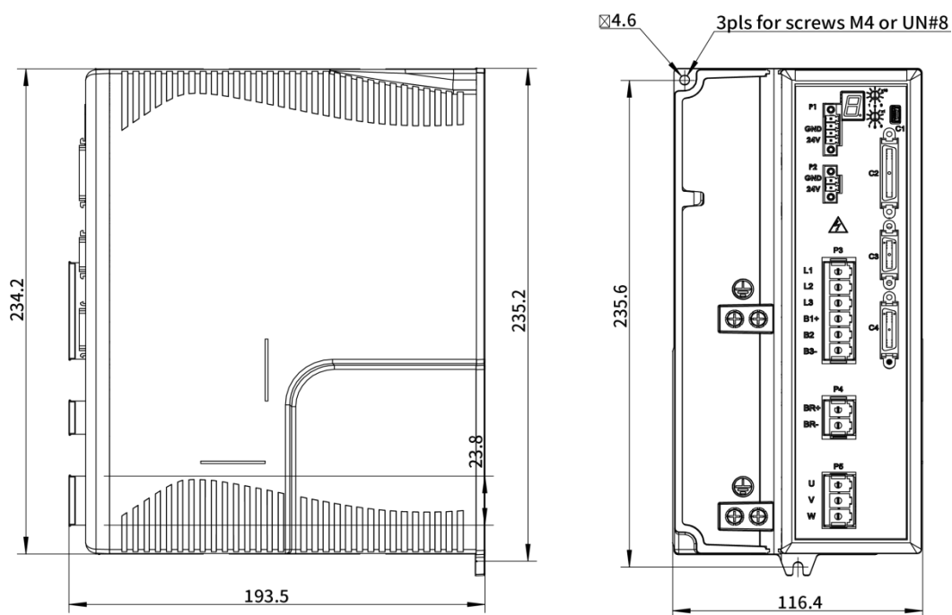
图 3-4 CDHD2S-012(高压) - 尺寸(mm)
