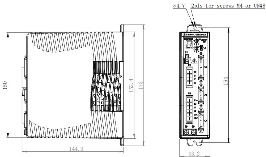
图 3-1 CDHD2S-003(中压 PN 机型) - 尺寸(mm)
