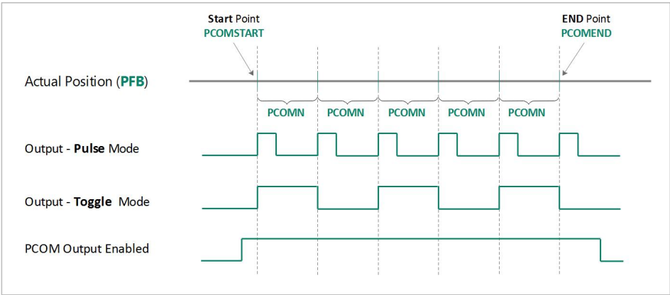
图 6-25 位置比较触发器输出-周期配置
