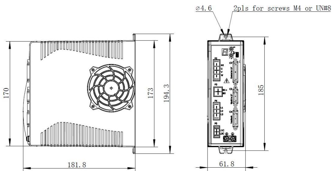
图 3-3 CDHD2S-010(中压 PN 机型) - 尺寸(mm)
