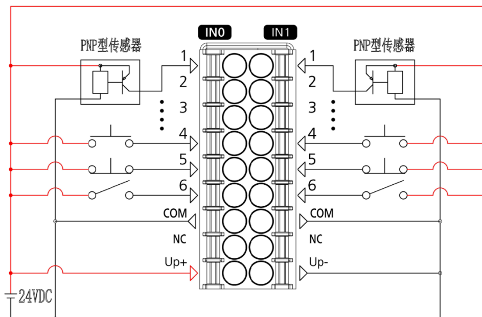
图 4-11 PNP 型传感器接线示意图
