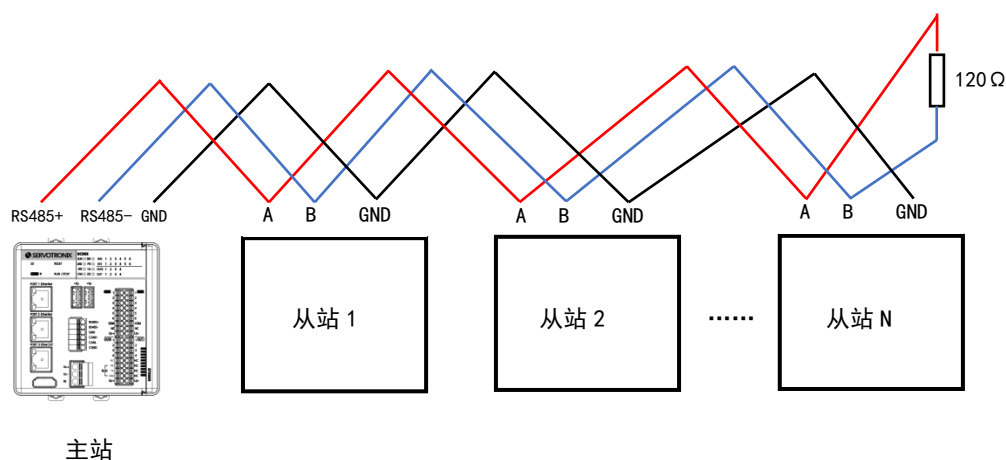
图 4-15 RS-485 菊花链拓扑结构示意图
