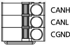
图 4-18 CAN 接口
