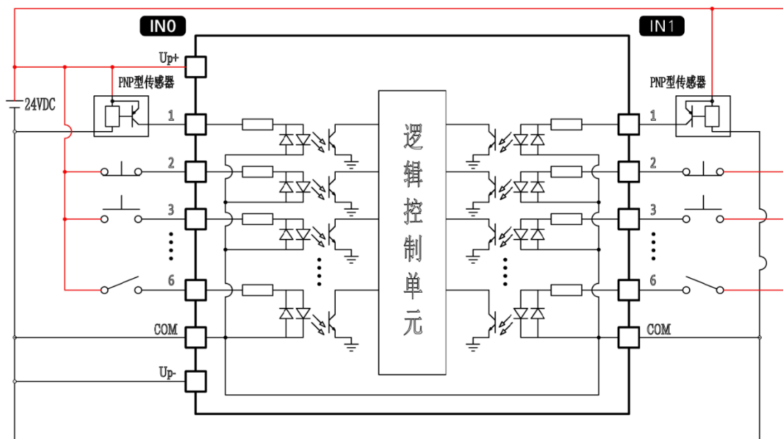
图 4-13 PNP 型传感器接线原理图
