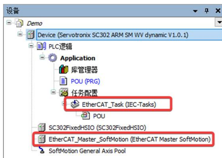
图 7-3 EtherCAT Master SoftMotion 添加成功
