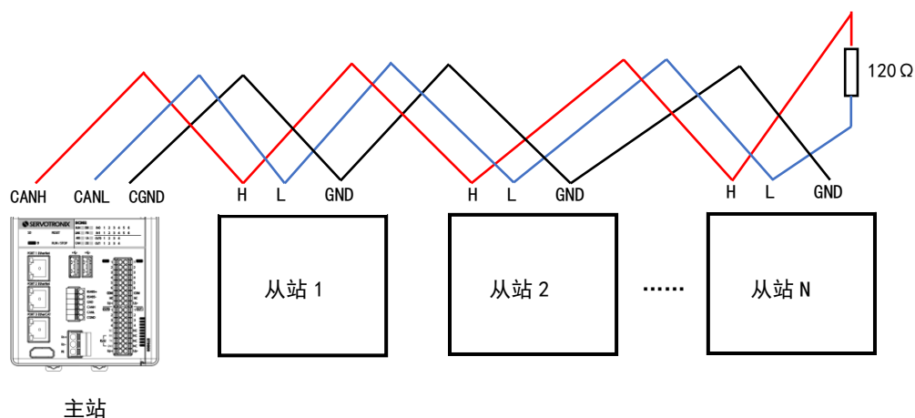
图 4-19 CAN 总线菊花链拓扑结构示意图
