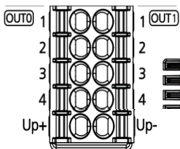
图 4-21 数字量输出接口
