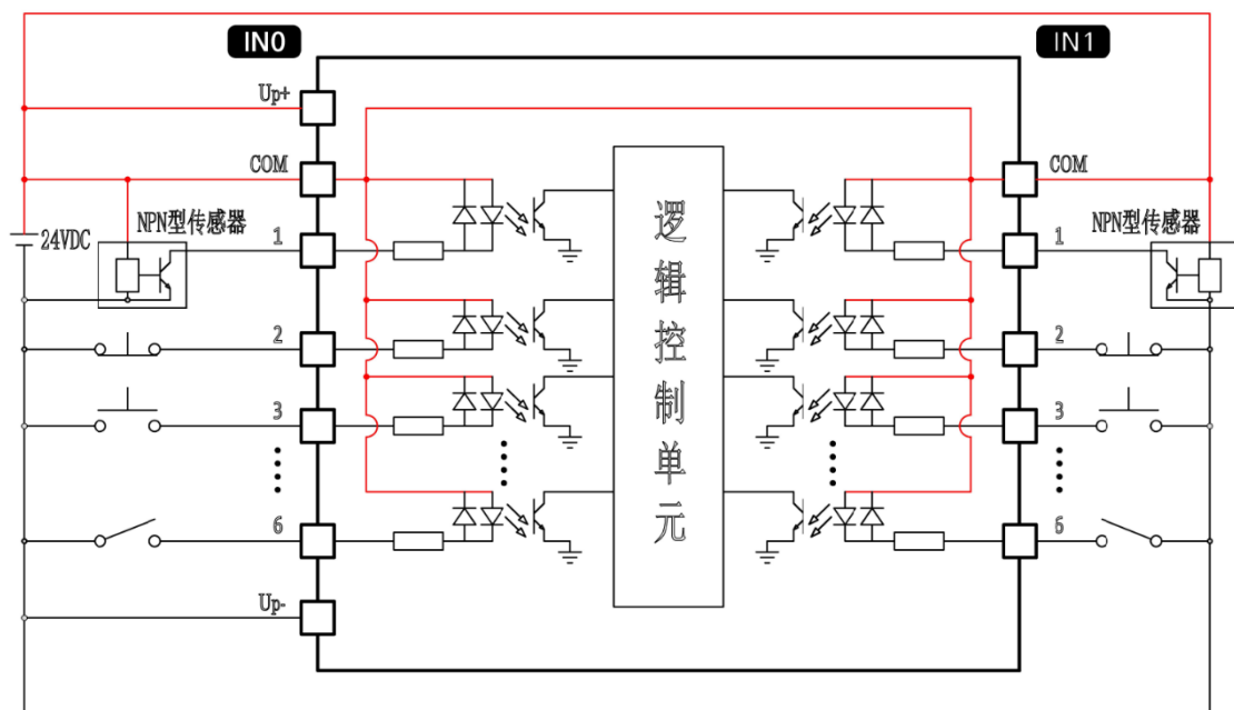
图 4-12 NPN 型传感器接线原理图
