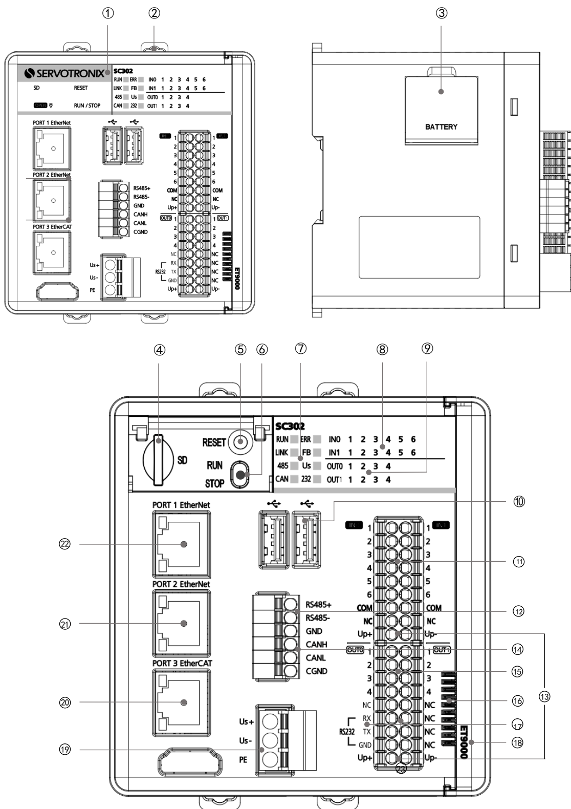
图 3-2 SC302 硬件接口
