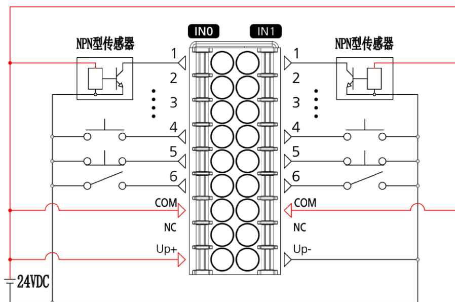
图 4-10 NPN 型传感器接线示意图
