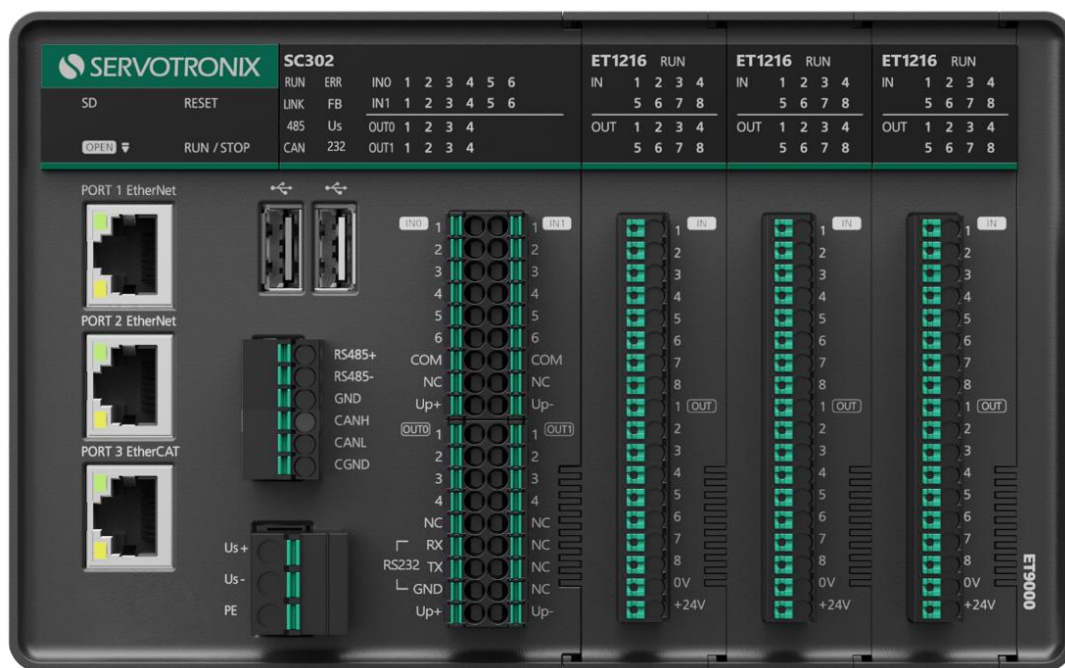
图 1-1 SC302 运动控制器搭配 ET 系列 I/O 模块组合图
