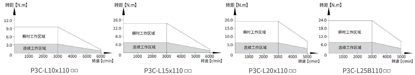
转矩特性图
