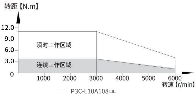
转矩特性图
