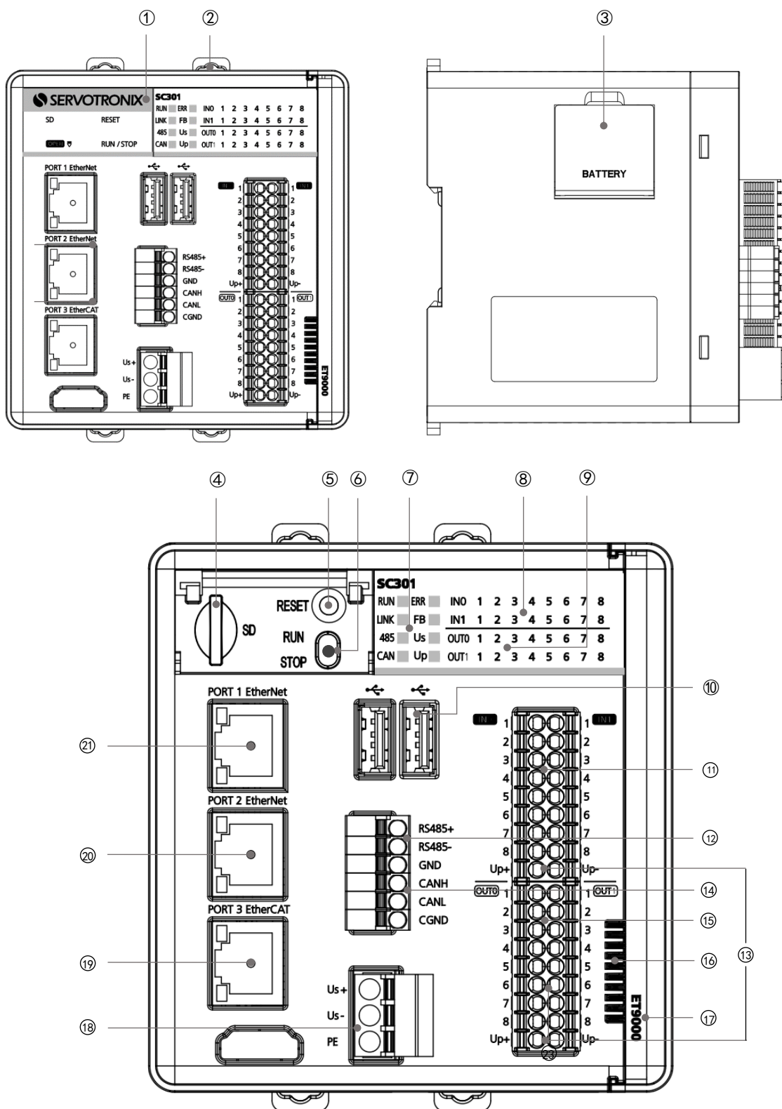
图 3-2 SC301 硬件接口
