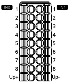
图 4-9 数字量输入接口
