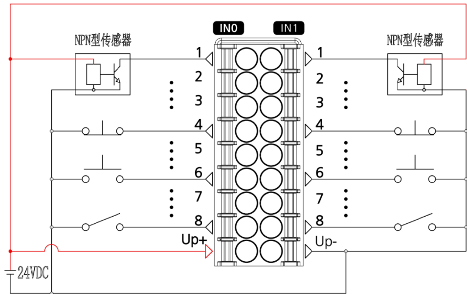
图 4-10 数字量输入接口接线示意图
