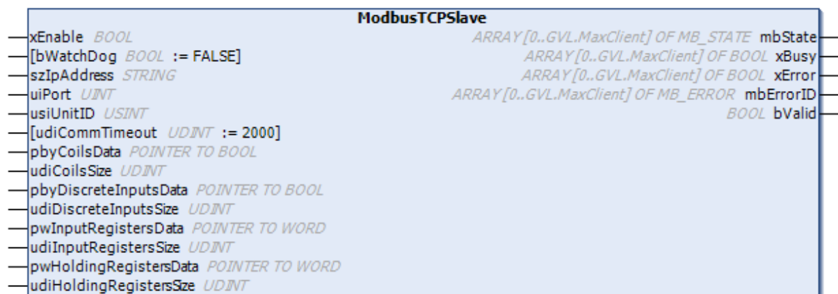
图 10-20 ModbusTCPSlave 指令图（多连接）
